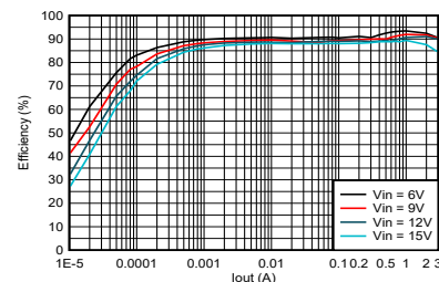
効率と出力電流との関係 (2.5MHz、1 \mu H、自動 PFM または PWM で V_O = 3.3V )
