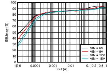
効率と出力電流との関係
