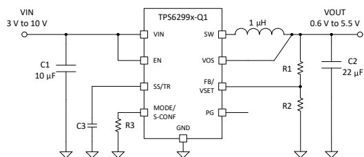
簡略回路図
