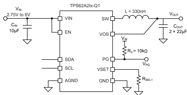
概略回路図 (TPS62A2Ix-Q1)
