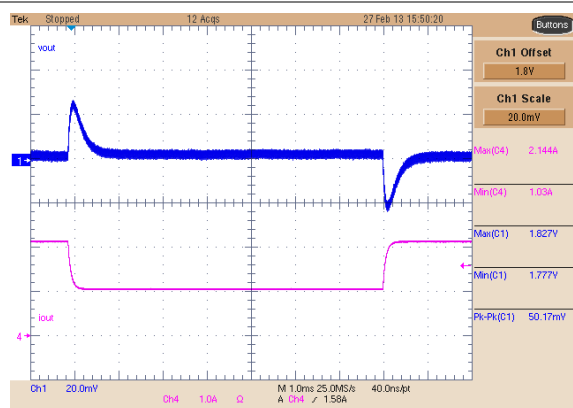
8-29. Buck 2 Dynamic Response, 1-A to 2-A Step
