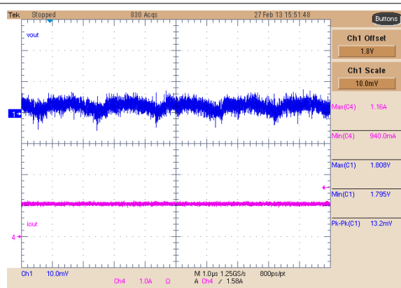
8-31. Buck 2 Ripple, 1-A Load
