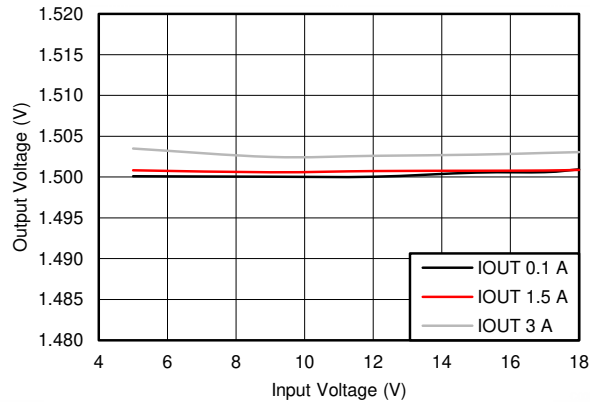
图 7-7. BUCK1, Line Regulation
