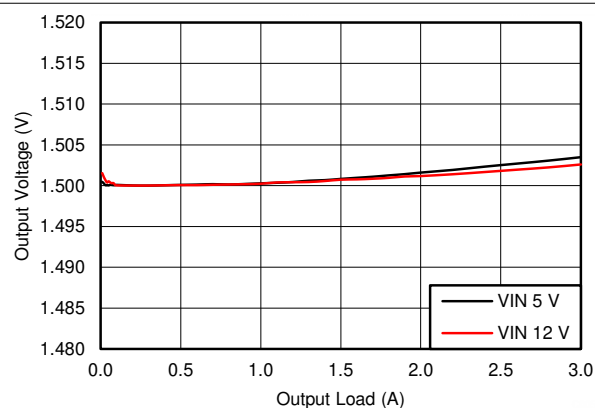
图 7-4. BUCK1 Load Regulation
