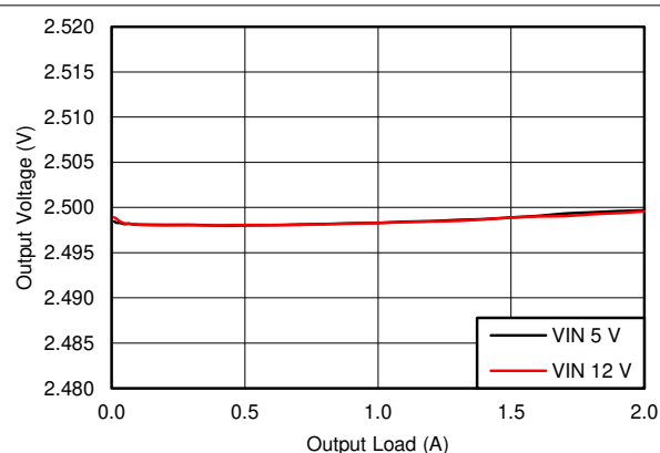
图 7-6. BUCK3 Load Regulation
