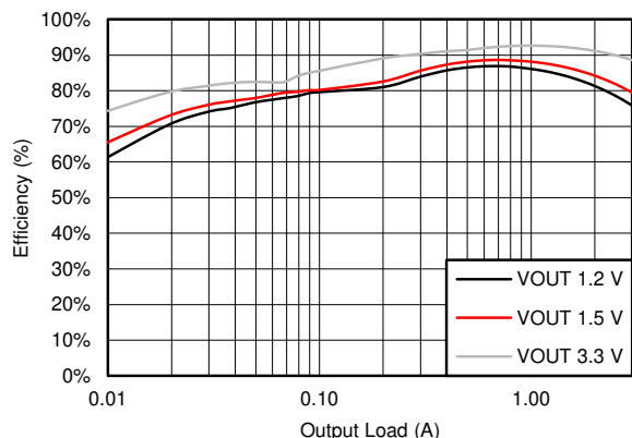
图 7-1. BUCK1 Efficiency
