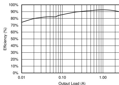
効率と出力負荷との関係
