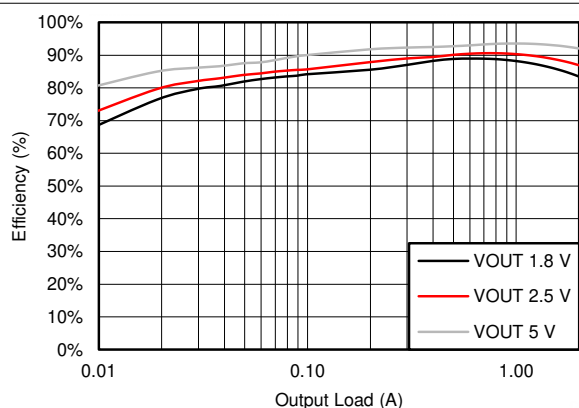
图 7-3. BUCK3 Efficiency
