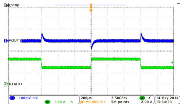
图 9-9. BUCK1, Load Transient, 1.5 to 2.25 A SR = 0.25 A/µs
