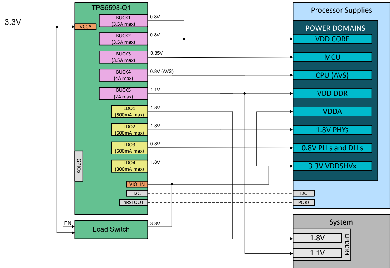
図 9-1. Example Power Map
