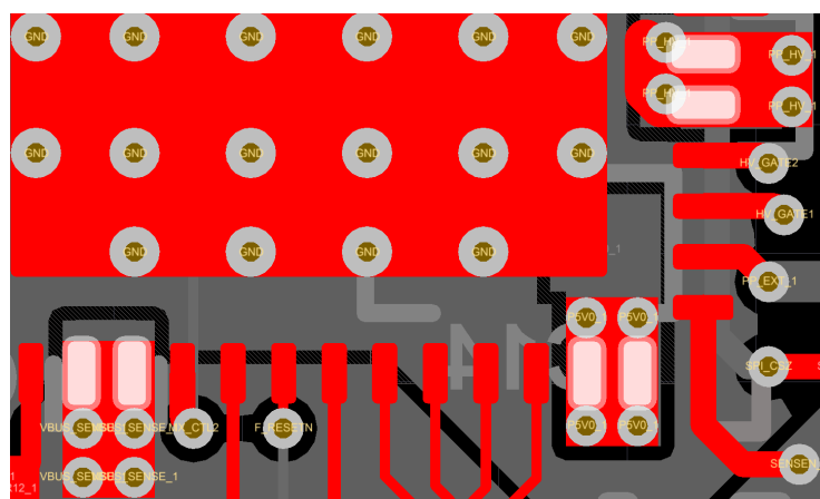
12-7. Top Polygonal Pours
