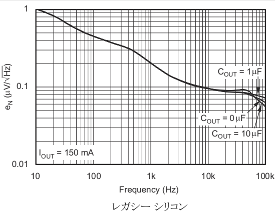
図 5-29. ノイズスペクトル密度 C_{NR} = 0.01\mu\text{F}
