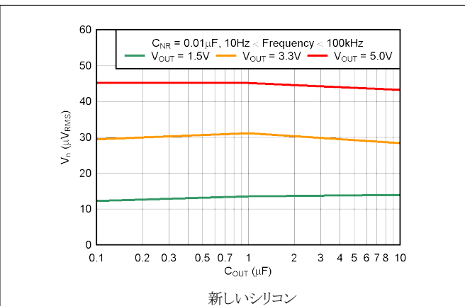
図 5-32. RMS ノイズ電圧と C_{OUT} との関係
