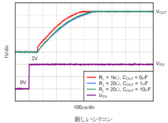
図 5-40. TPS73233 のターンオン応答
