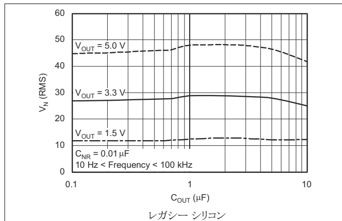
図 5-31. RMS ノイズ電圧と C_{OUT} との関係
