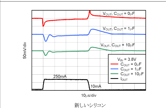
図 5-36. TPS73233 の負荷過渡応答
