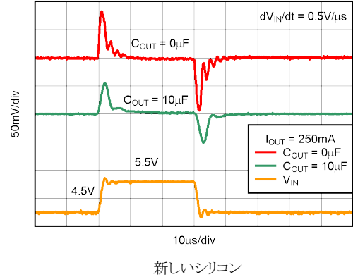
図 5-38. TPS73233 のライン過渡応答
