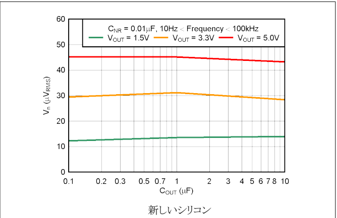
図 5-32. RMS ノイズ電圧と C_{OUT} との関係
