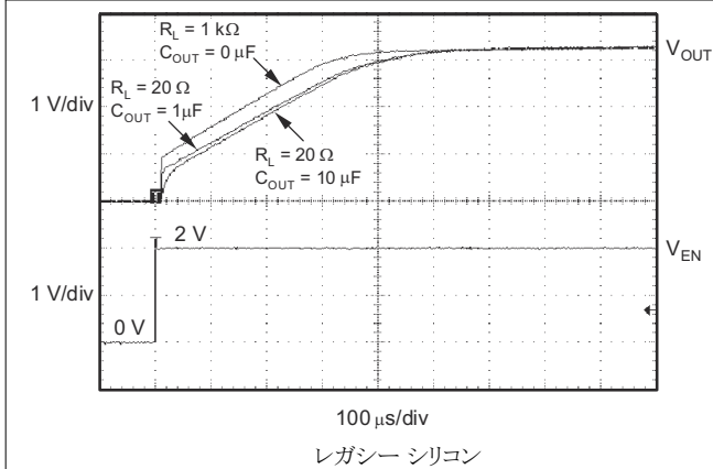
図 5-39. TPS73233 のターンオン応答
