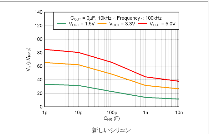
図 5-34. RMS ノイズ電圧と C_{NR} との関係
