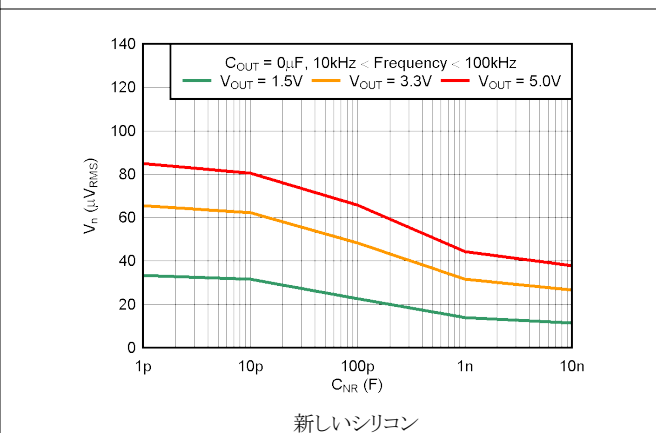
図 5-34. RMS ノイズ電圧と C_{NR} との関係
