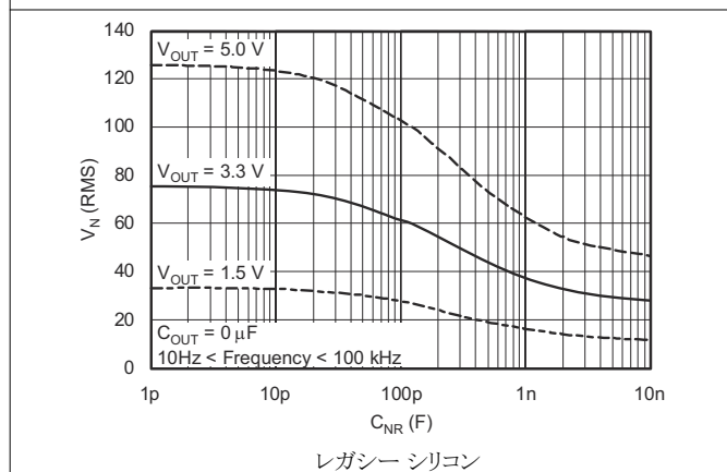
図 5-33. RMS ノイズ電圧と C_{NR} との関係
