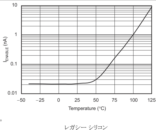
図 5-45. I_{ENABLE} VS 温度
