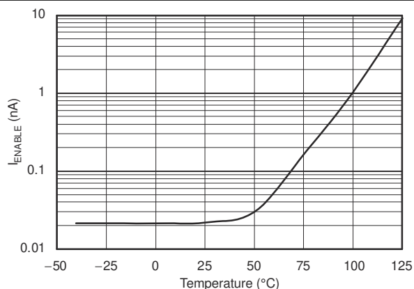
図 5-24. I_{ENABLE} VS 温度
