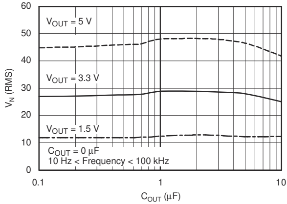
図 5-17. RMS ノイズ電圧と C_{OUT} との関係
