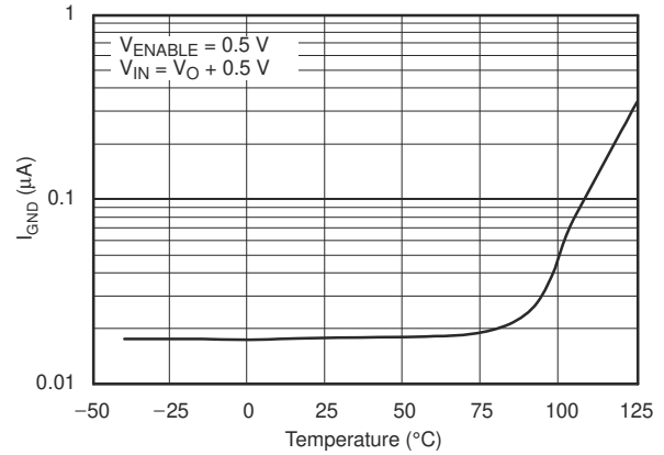
図 5-10. シャットダウン時のグランドピンの電流と温度との関係
