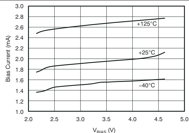
图 5-24. I_{BIAS} vs V_{BIAS} and V_{OUT} (legacy chip)
