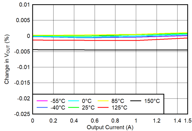
図 7-8. Load Regulation
