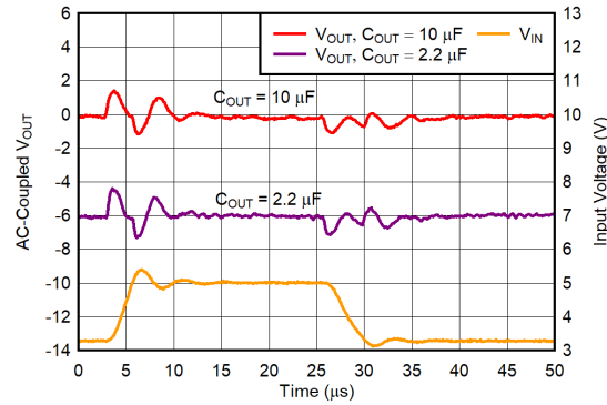
図 7-6. V_{BIAS} Line Transient
