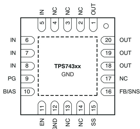
図 4-1. RGW PACKAGE 5 × 5 QFN-20 (TOP VIEW)
