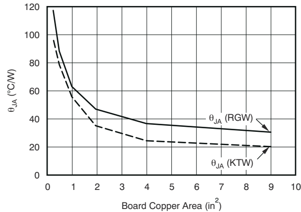
図 7-9. \theta_{JA} vs Board Size
