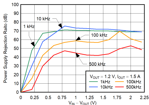
图 5-19. V_{IN} PSRR vs (V_{IN} - V_{OUT}) (new chip)
