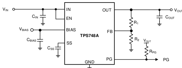
図 7-1. 代表的な ADJ 電圧アプリケーション
