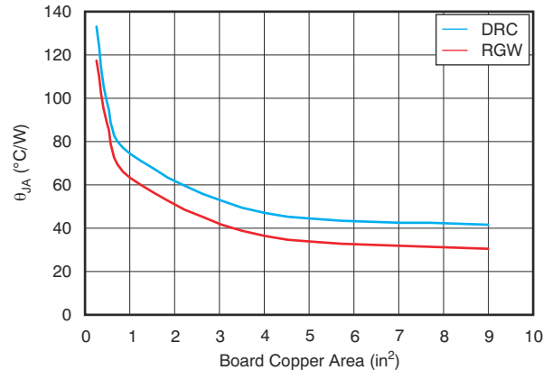
図 7-3. R_{\theta JA} と基板サイズとの関係
