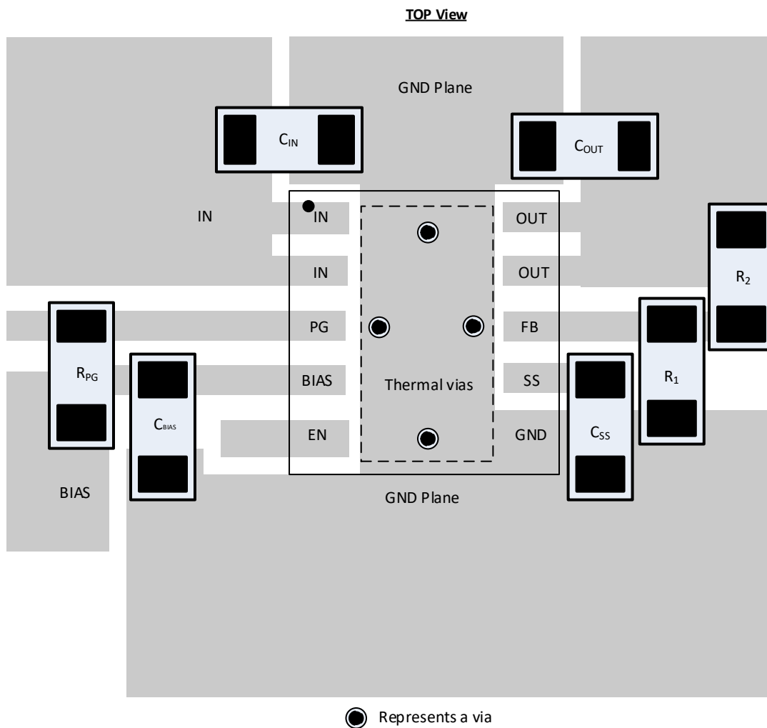
図 7-4. レイアウト例
