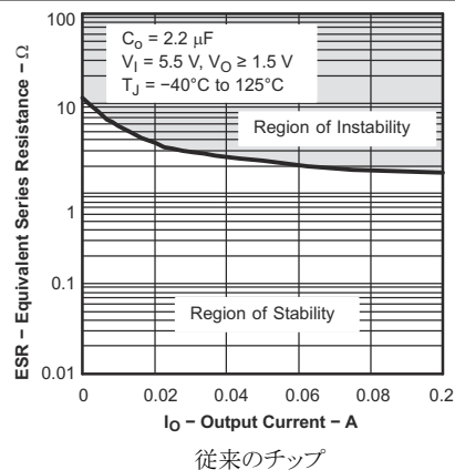
図 5-34. 安定等価直列抵抗 (ESR) の標準的な領域と出力電流との関係
