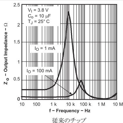
図 5-12. 出力インピーダンス 対 周波数
