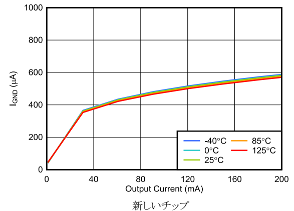
図 5-6. TPS793-Q1 接地電流と接合部温度との関係
