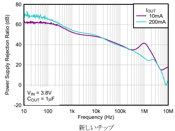
図 5-20. TPS793-Q1 リップル除去と周波数との関係
