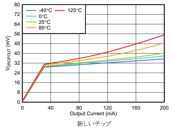
図 5-30. ドロップアウト電圧と出力電流との関係
