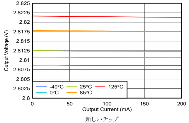
図 5-2. TPS793-Q1 の出力電圧と出力電流との関係
