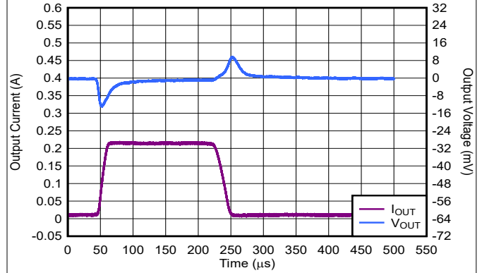
図 5-26. TPS79328 の負荷過渡応答
