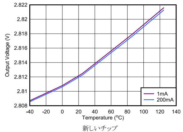
図 5-4. TPS793-Q1 の出力電圧と接合部温度との関係
