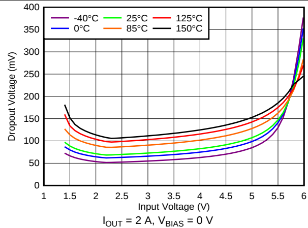
I_{OUT} = 2\text{ A} , V_{BIAS} = 0\text{ V}
