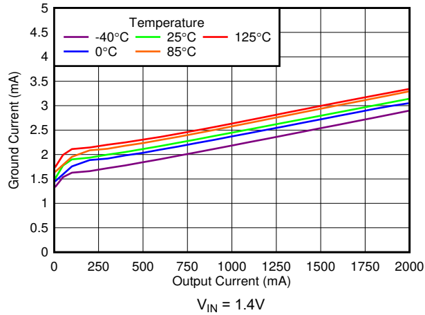
図 5-19. グランド電流と出力電流との関係
