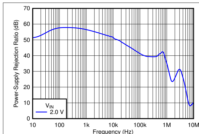
図 7-3. PSRR と周波数との関係
