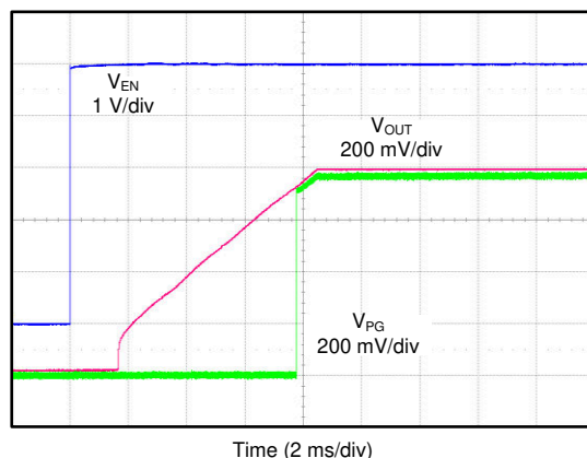
図 5-35. スタートアップ ( SS\_CTRL = V_{IN} 、 C_{NR/SS} = 1\mu\text{F} )
