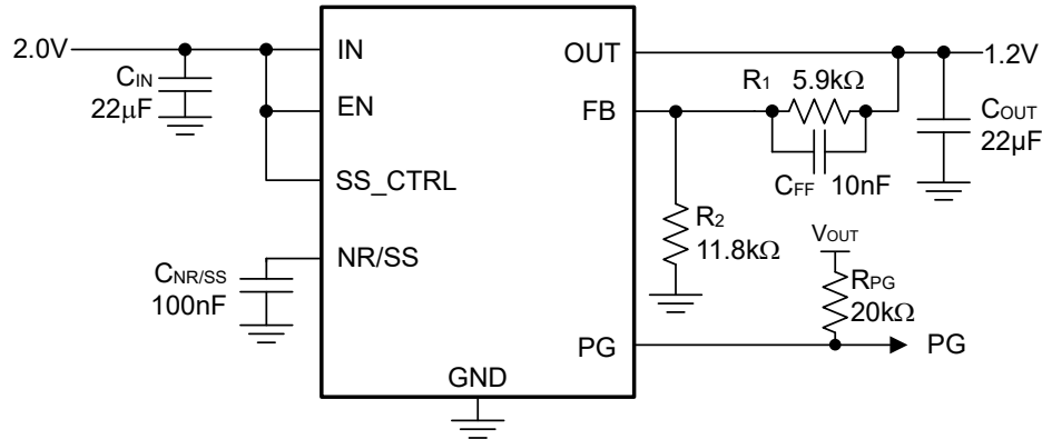
図 7-2. アプリケーションの例
