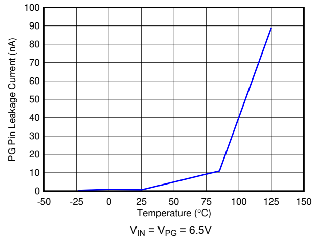
図 5-24. PG リーク電流と温度との関係
