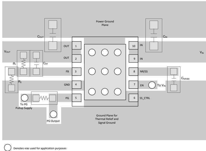
図 7-5. TPS7A92 のレイアウト例
