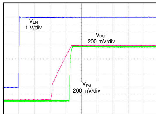
図 5-32. スタートアップ ( SS\_CTRL = \text{GND} , C_{NR/SS} = 0\text{nF} )
