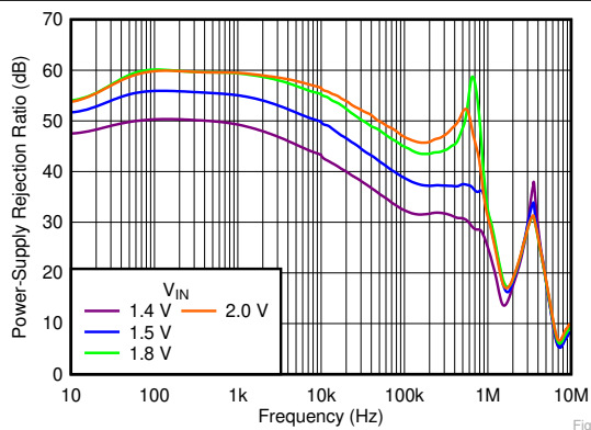
図 5-1. PSRR と周波数および入力電圧との関係
