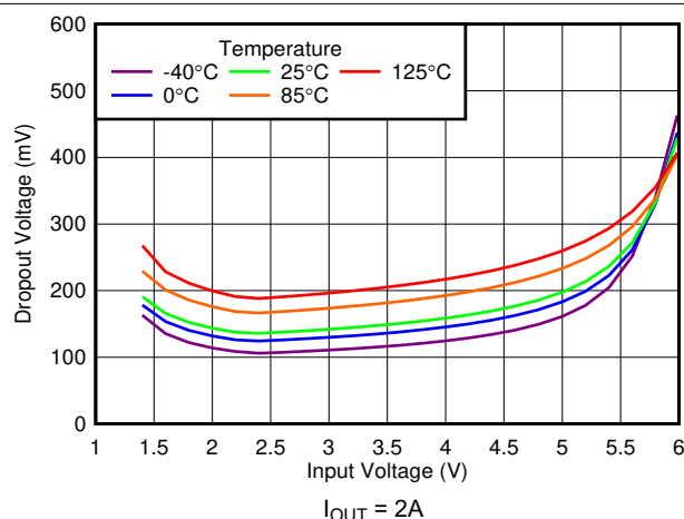
図 5-15. ドロップアウト電圧と入力電圧との関係
