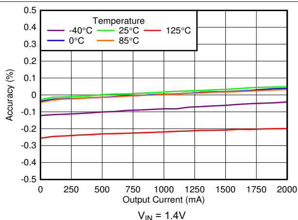
図 5-16. ロードレギュレーション
