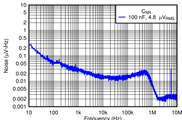
図 7-4. 出力ノイズと周波数との関係
