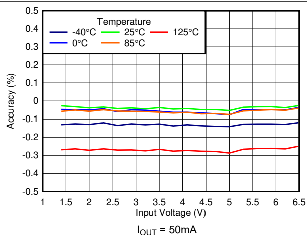
図 5-17. ラインレギュレーション
