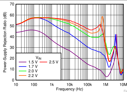
図 5-2. PSRR と周波数および入力電圧との関係
