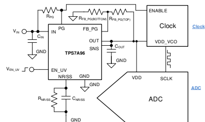
代表的なアプリケーション回路
