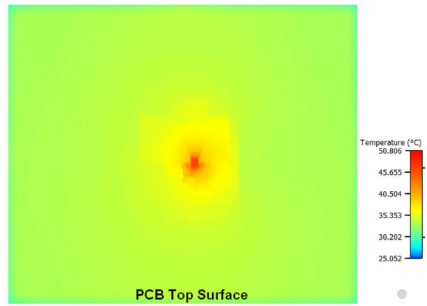
☒ 8-24. TPS7A96EVM-106 PCB Thermal Gradient
