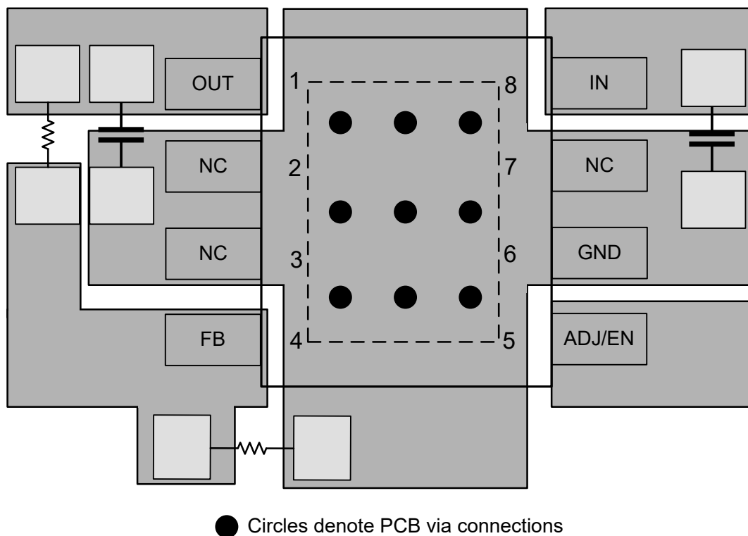
図 7-10. DDA Package Layout Example
