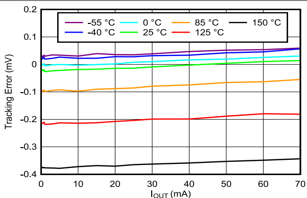
図 5-2. Tracking Error vs Output Current
