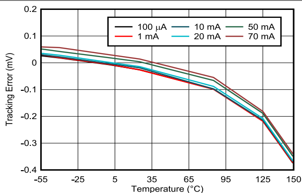
図 5-1. Tracking Error vs Ambient Temperature
