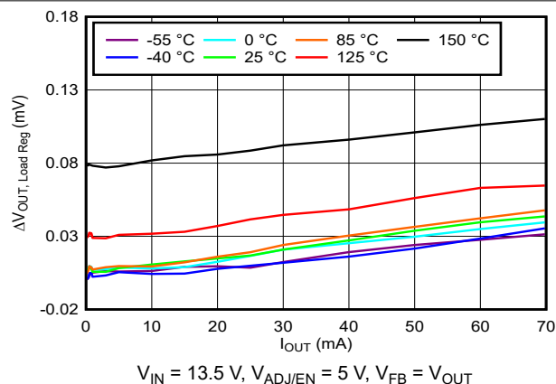
図 5-7. Load Regulation
