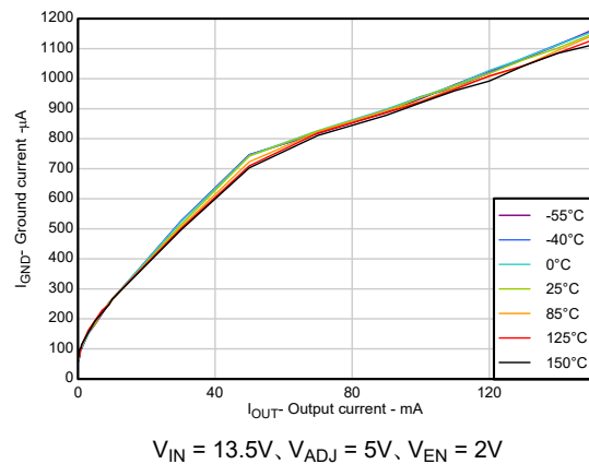
図 5-12. グランド電流と出力電流との関係
