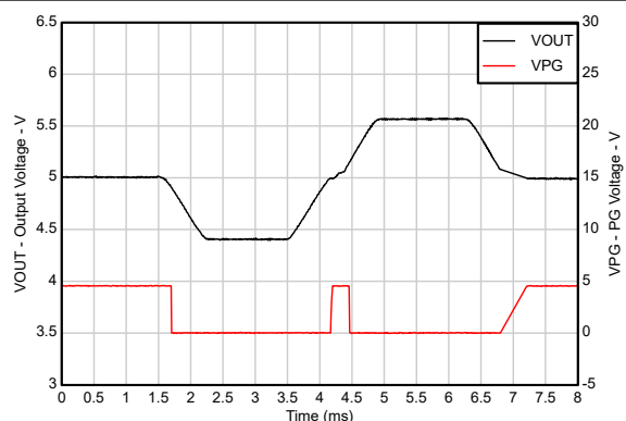
図 5-32. ライン過渡応答
