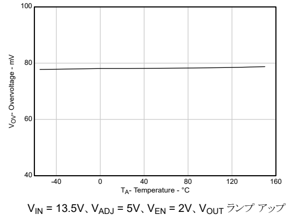
図 5-22. 過電圧トリップスレッシュホールドと周囲温度との関係
