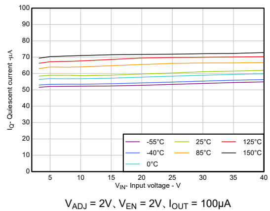
図 5-10. 静止電流と入力電圧との関係
