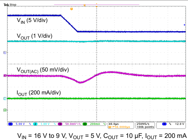
图 5-18. Line Transient
