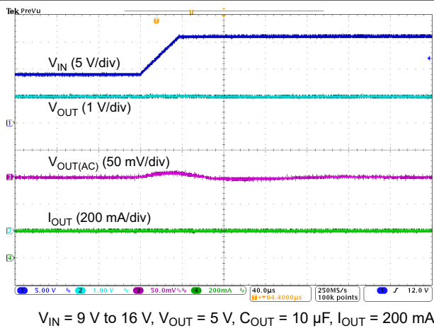
图 5-17. Line Transient
