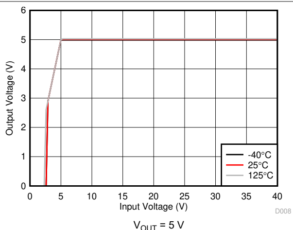
図 5-8. Output Voltage vs Input Voltage
