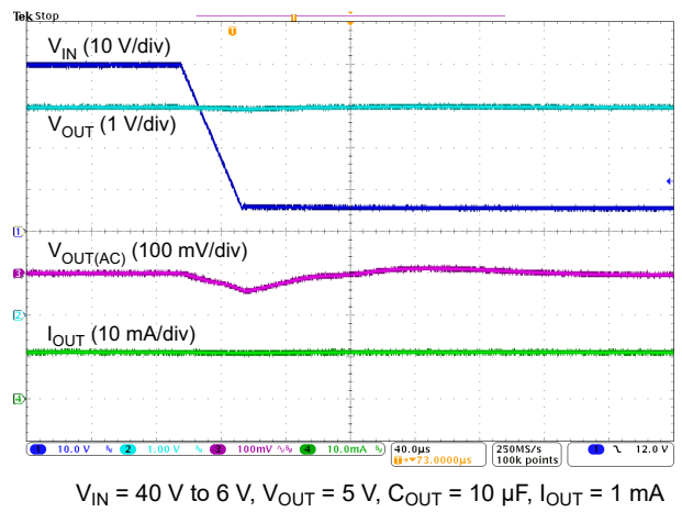
图 5-16. Line Transient
