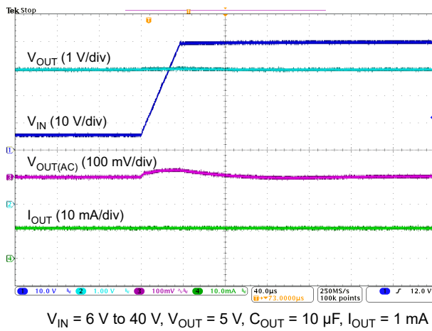
图 5-15. Line Transient
