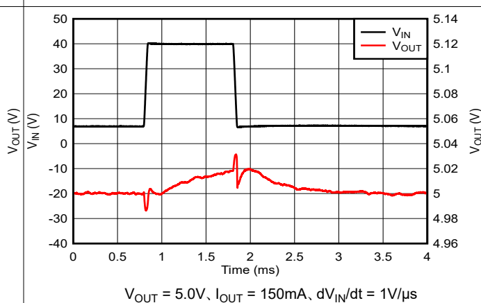
図 7-7. V_{IN} ライン過渡応答 (7V~40V)
