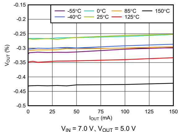
図 5-10. V_{OUT} の精度と I_{OUT} との関係
