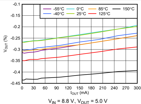
図 5-11. V_{OUT} の精度と I_{OUT} との関係
