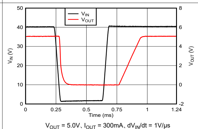
図 5-36. ブラウンアウト過渡応答 (40V~1.7V)
