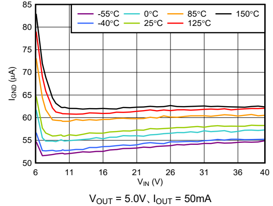
図 5-14. I_{GND} と V_{IN} との関係
