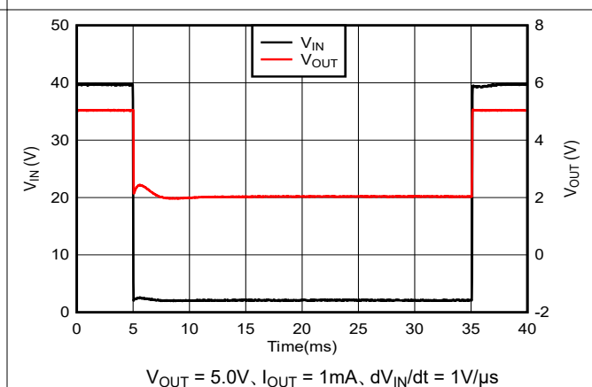
図 5-34. ブラウンアウト過渡応答 (40V~2.1V)
