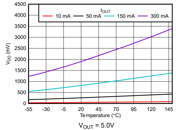
図 5-16. ドロップアウトと温度との関係
