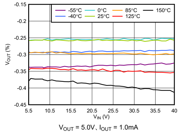
図 5-8. V_{OUT} の精度と V_{IN} との関係
