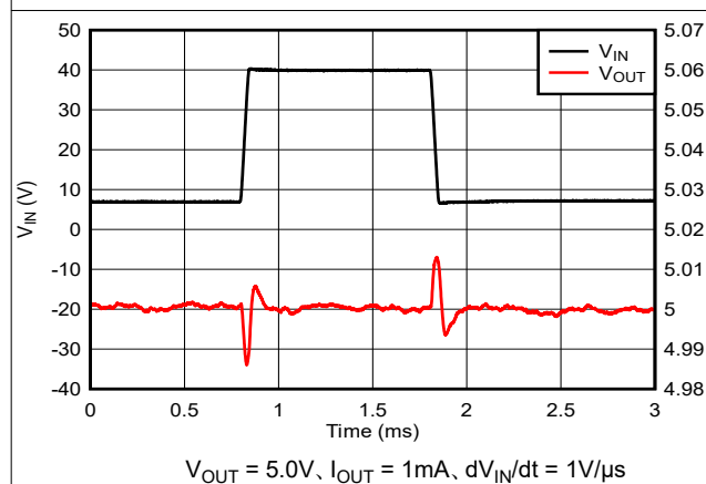
図 7-6. V_{IN} ライン過渡応答 (7V~40V)
