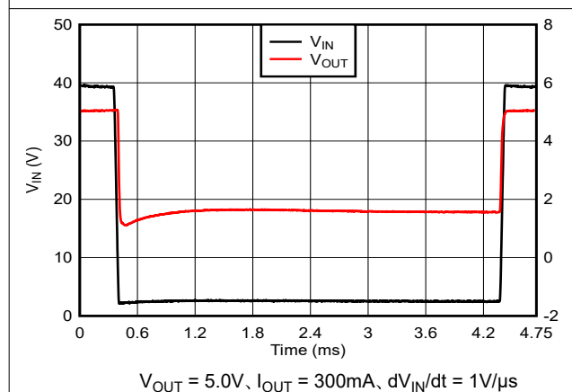
図 5-35. ブラウンアウト過渡応答 (40V~2.5V)
