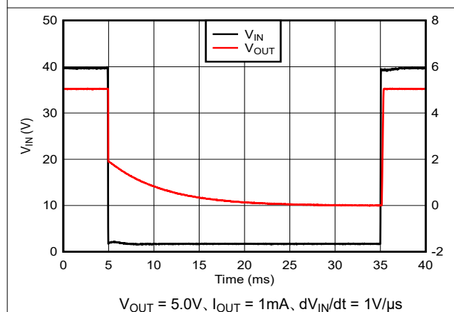
図 5-33. ブラウンアウト過渡応答 (40V~1.7V)
