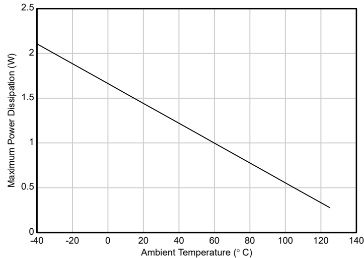
図 7-3. TPS7E71 (DRV) 許容消費電力
