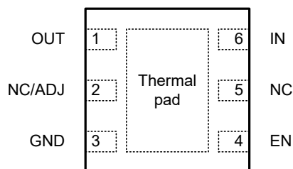
図 4-2. DRV パッケージ (固定/可変)、6 ピン WSON (上面図)
