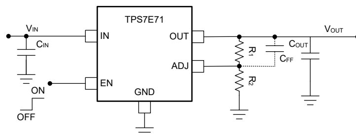
図 7-5. TPS7E71 可変 LDO レギュレータのプログラミング
