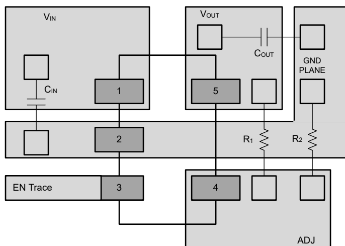
図 7-11. TPS7E71、DBV パッケージのレイアウト例
