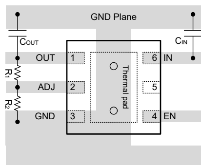
図 7-12. TPS7E71、DRV パッケージのレイアウト例
