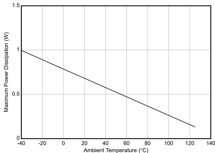
図 7-2. TPS7E71 (DBV) 許容消費電力
