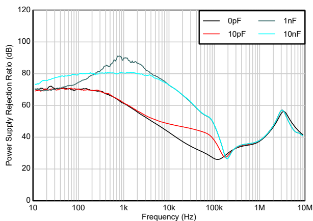
図 5-22. リップル除去と周波数、 C_{FF} との関係
