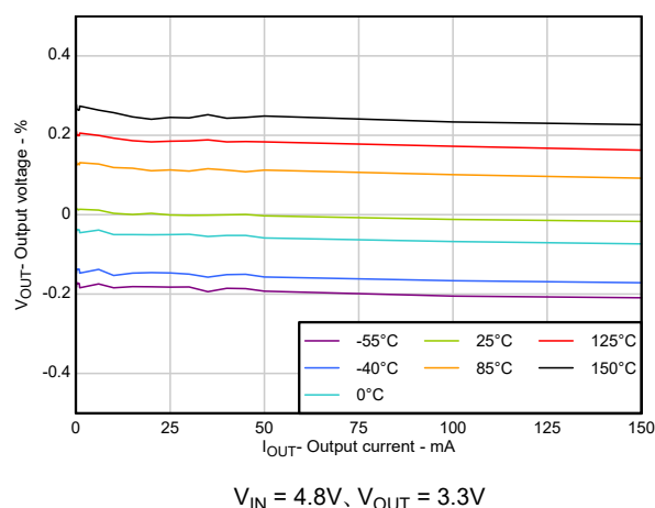
V_{OUT} の精度と I_{OUT} との関係
