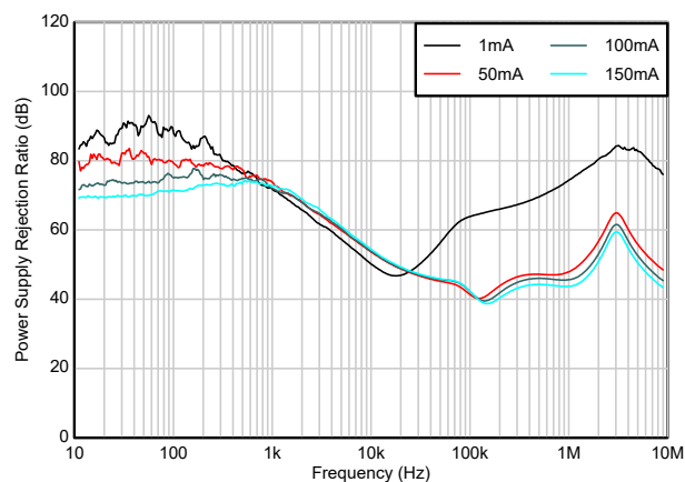
図 5-21. リップル除去と周波数、出力電流との関係
