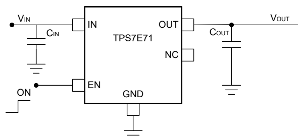
図 7-4. TPS7E71 代表的なアプリケーション回路 (固定電圧バージョン)
