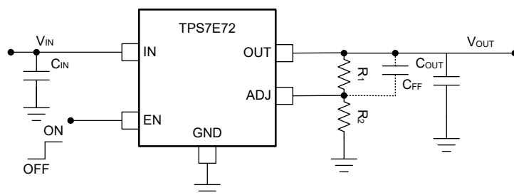
図 7-5. TPS7E72 の可変 LDO レギュレータのプログラミング
