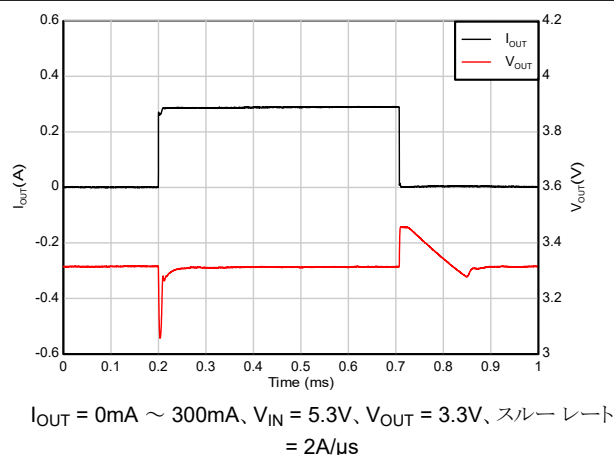
図 5-35. 負荷過渡応答
