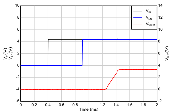
図 7-6. ライト トランジェント
