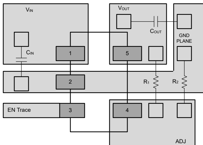
図 7-11. TPS7E72 (DBV) パッケージのレイアウト例
