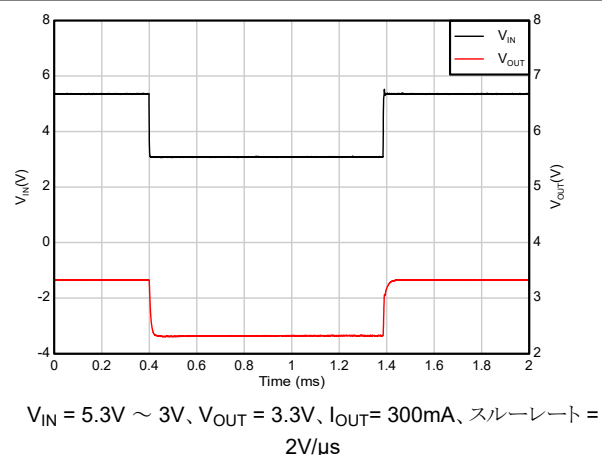
図 5-38. ドロップアウトからの回復
