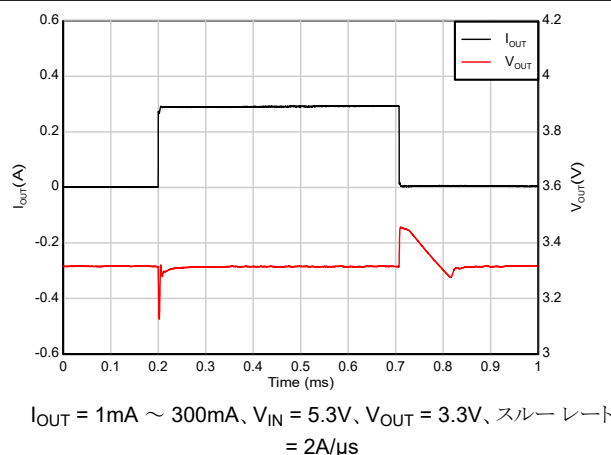
図 5-36. 負荷過渡応答
