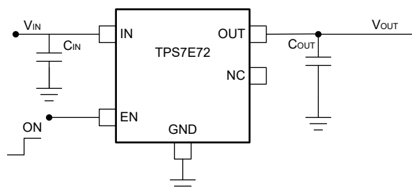
図 7-4. TPS7E72 の代表的なアプリケーションの回路 (固定電圧バージョン)
