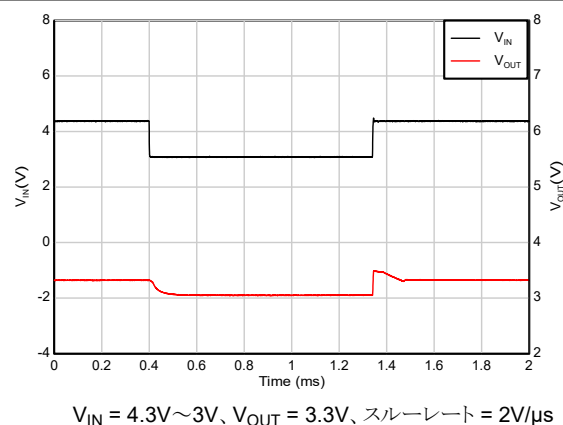
図 5-37. ドロップアウトからの回復
