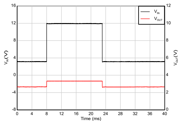
図 5-32. ライン トランジェント
