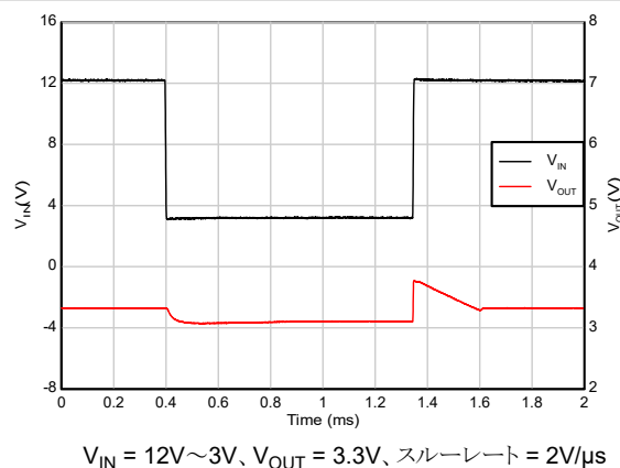
図 5-39. ドロップアウトからの回復
