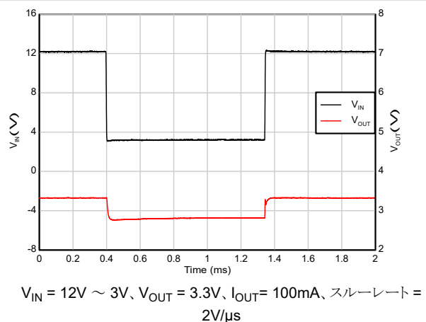
図 5-40. ドロップアウトからの回復
