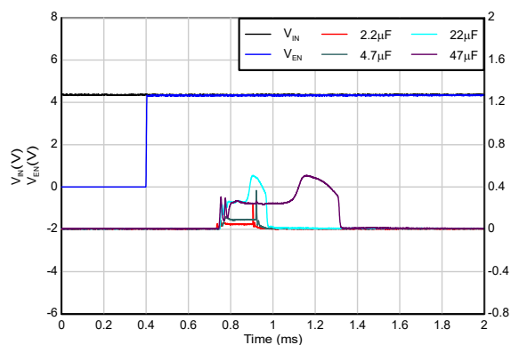
図 5-43. スタートアップ突入電流
