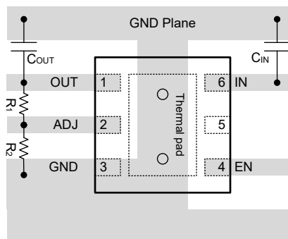
図 7-12. TPS7E72 (DRV) パッケージのレイアウト例
