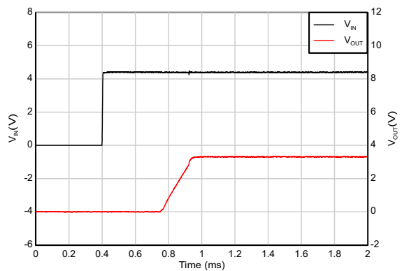
図 7-8. シーケンシングありの起動 (IN の後に EN)
