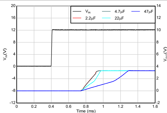
図 5-48. IN と EN を接続した場合の起動
