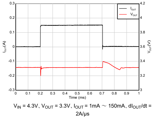
図 5-43. 負荷過渡応答 (1mA~150mA)
