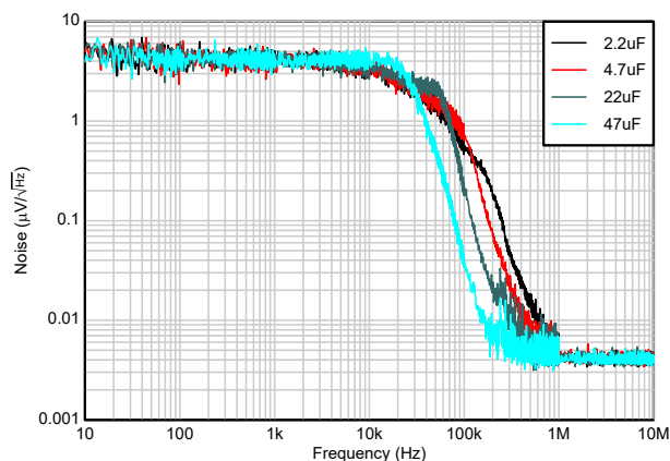
図 5-25. ノイズと C_{OUT} との関係
