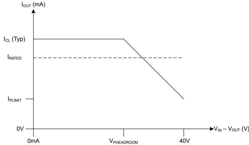
図 6-6. 電力制限
