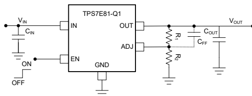
図 3-1. 代表的なアプリケーション
