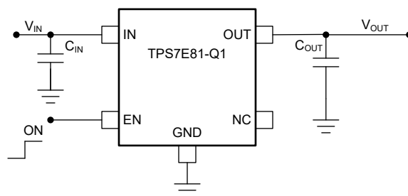
図 7-5. 代表的なアプリケーションの回路 (固定電圧バージョン)
