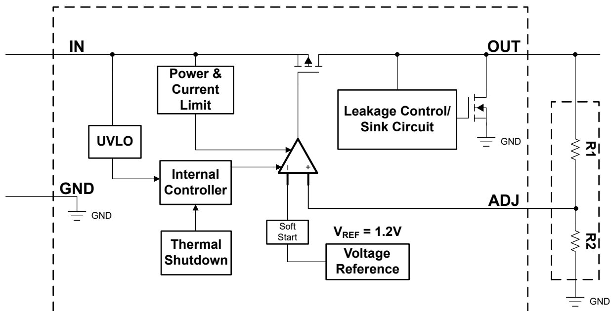
図 6-3. 機能ブロック図：可変バージョン (EN 機能なし)
