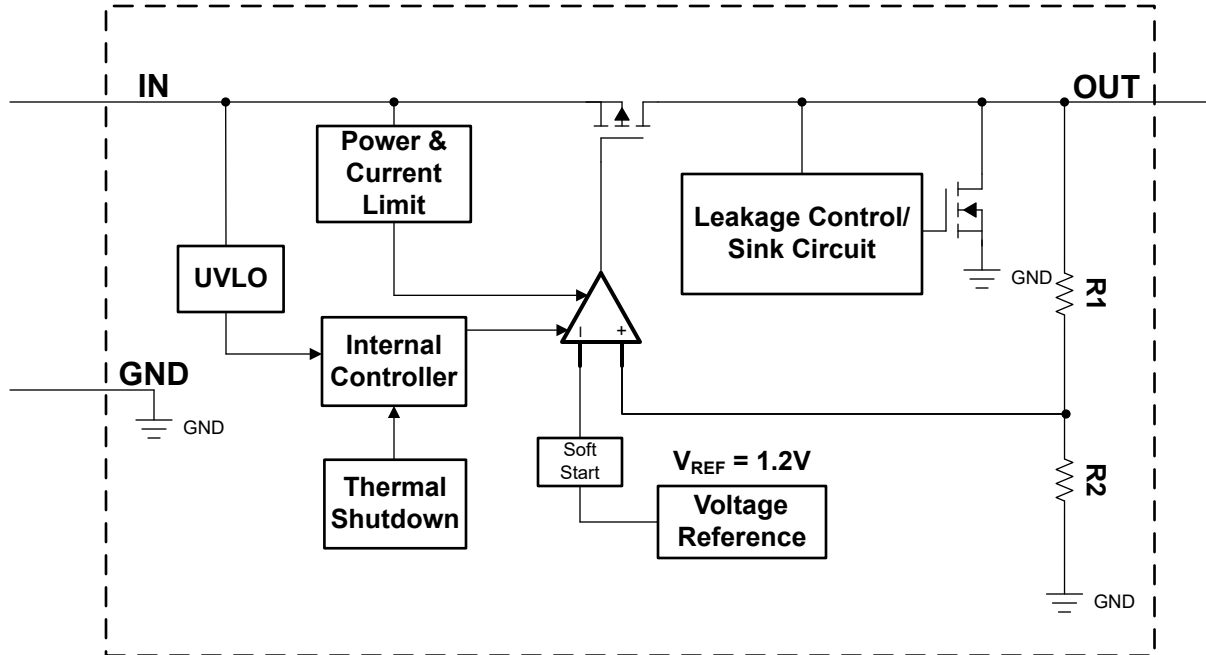
図 6-4. 機能ブロック図：固定バージョン (EN 機能なし)
