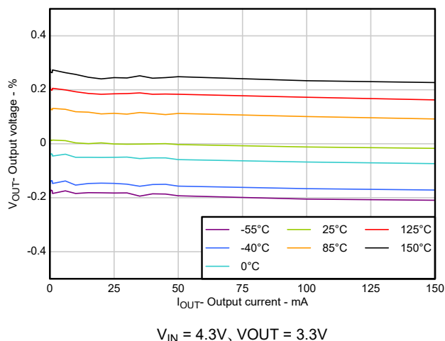
図 2-1. V_{OUT} の精度と I_{OUT} との関係
