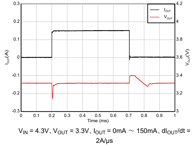
図 5-42. 負荷過渡応答 (0mA~150mA)
