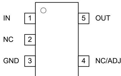
図 4-4. DBV パッケージ、[A バージョン、EN なし] (固定/可変)、5 ピン SOT-23 (上面図)
