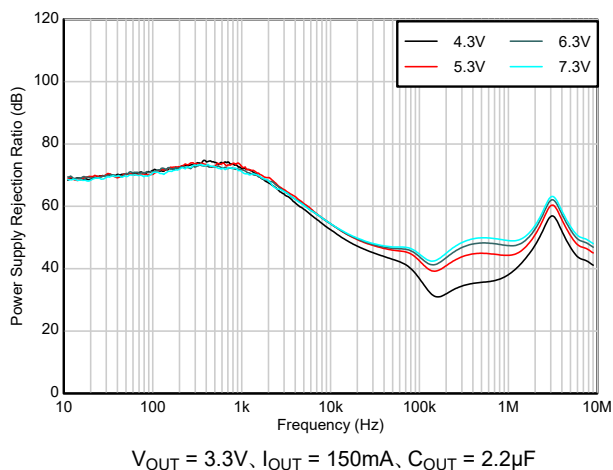
図 5-20. PSRR と V_{IN} との関係
