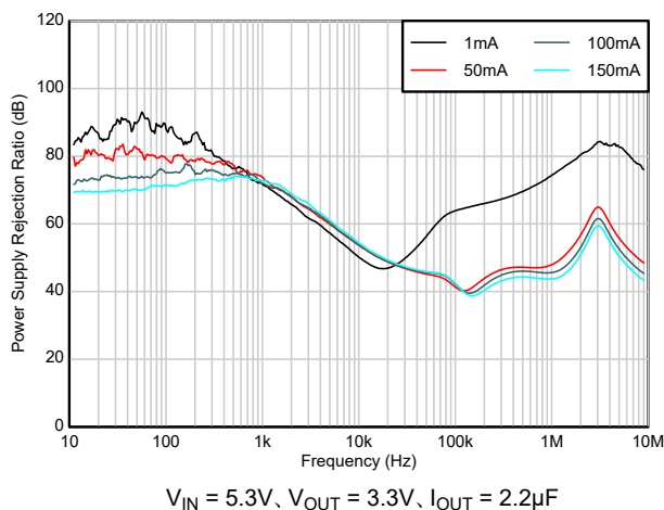
図 5-19. PSRR と I_{OUT} との関係
