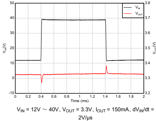
図 5-41. ライン過渡応答 (12V ~ 40V)
