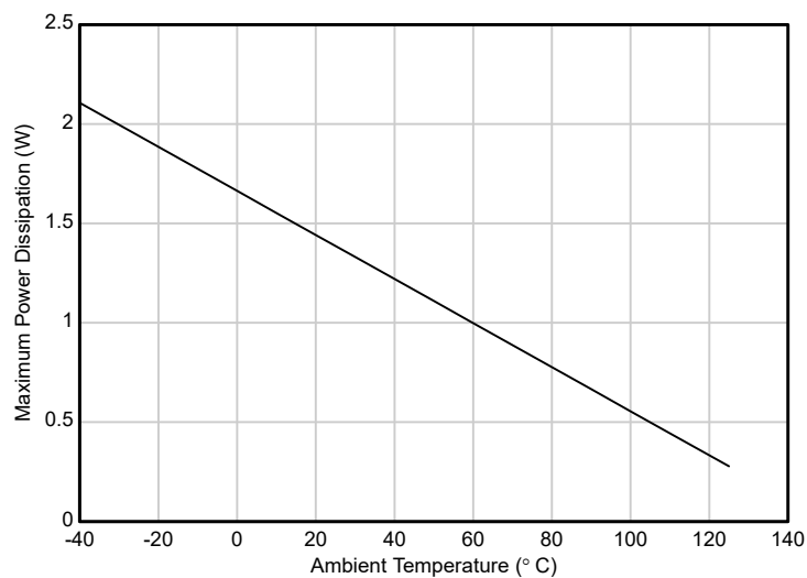
図 7-3. TPS7E81-Q1 (DRV) 許容消費電力
