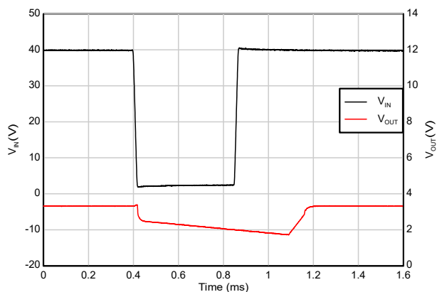
図 5-50. ブラウンアウトからの回復 (40V ~ 2V)
