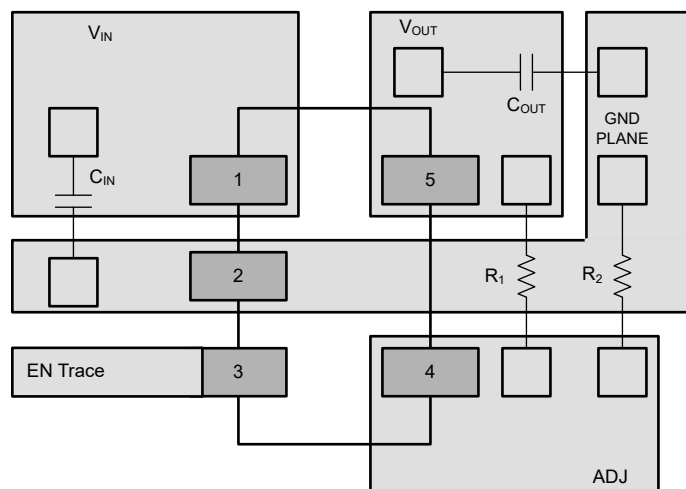
図 7-20. DBV パッケージのレイアウト例
