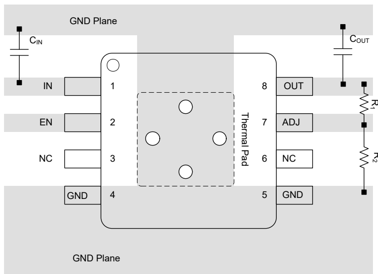
図 7-19. DGN パッケージのレイアウト例
