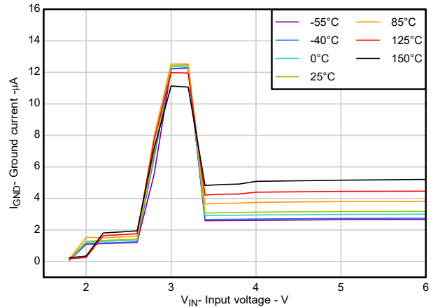
図 5-8. I_{GND} と V_{IN} との関係
