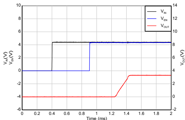
図 5-32. シーケンスによる起動 ( V_{IN} 後の EN)
