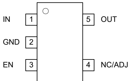
図 4-3. DBV パッケージ (固定/可変)、5 ピン SOT-23 (上面図)
