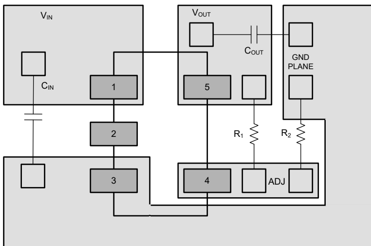
図 7-21. DBV-A (EN 機能なし) パッケージのレイアウト例
