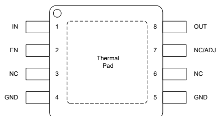
図 4-5. DGN パッケージ (固定/可変)、8 ピン HVSSOP (上面図)
