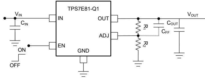
図 7-6. 可変 LDO レギュレータのプログラミング
