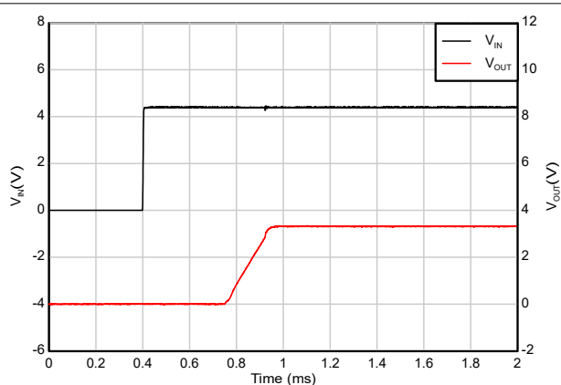
図 5-27. スタートアップと C_{OUT} との関係
