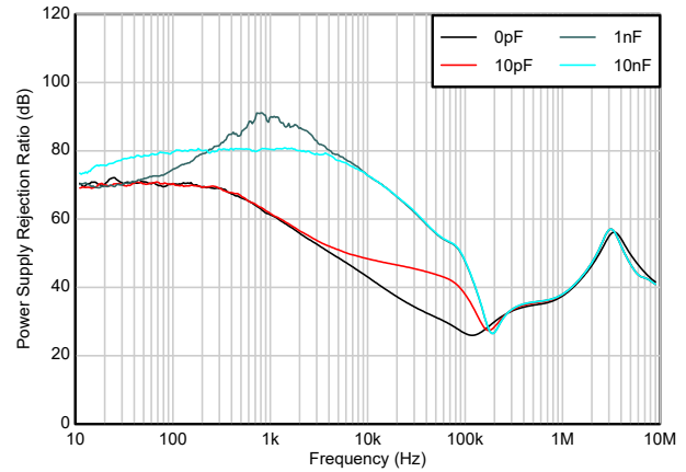
図 5-22. PSRR と C_{FF} との関係
