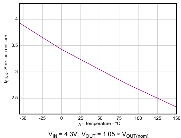
図 5-16. 出力オンのシンク電流 ( I_{SINK} ) と温度との関係
