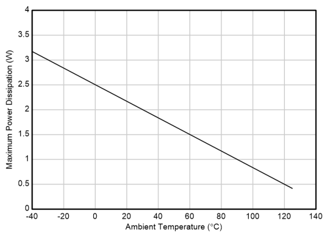
図 7-4. TPS7E81-Q1 (DGN) 許容消費電力
