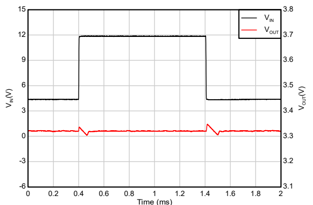
図 5-38. ライン過渡応答 (4.3V ~ 12V)
