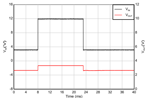
図 5-49. コールドクランク回復
