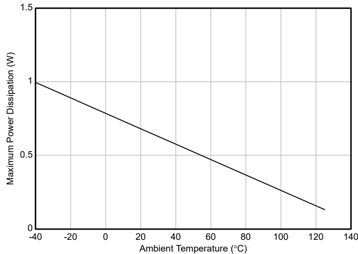
図 7-2. TPS7E81-Q1 (DBV) 許容消費電力
