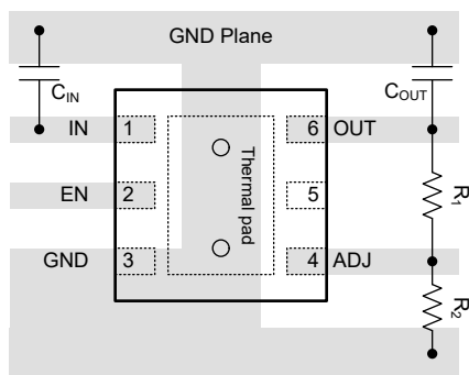
図 7-22. DRV パッケージのレイアウト例
