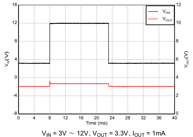
図 5-48. コールドクランク回復
