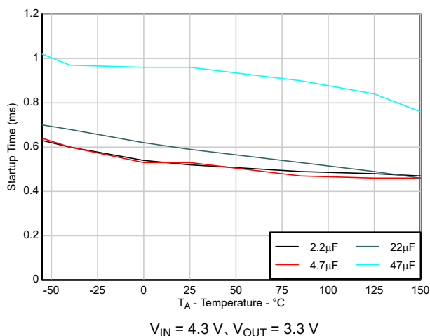
図 5-18. スタートアップタイムと C_{OUT} との関係
