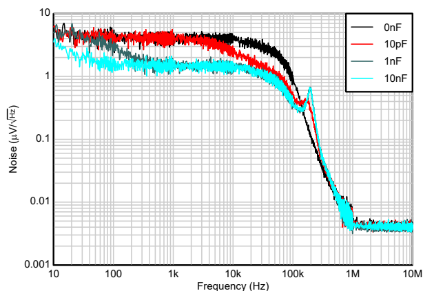
図 5-26. ノイズと C_{FF} との関係
