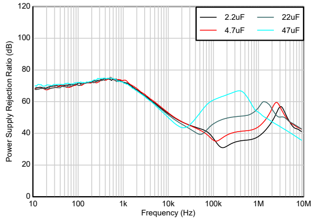
図 5-21. PSRR と C_{OUT} との関係
