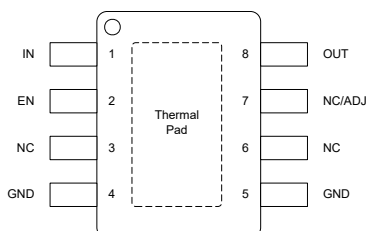
図 4-5. DGN パッケージ (固定/可変)、8 ピン HVSSOP (上面図)
