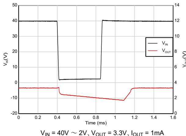
図 7-16. ブラウンアウトからの回復 (40V ~ 2V)
