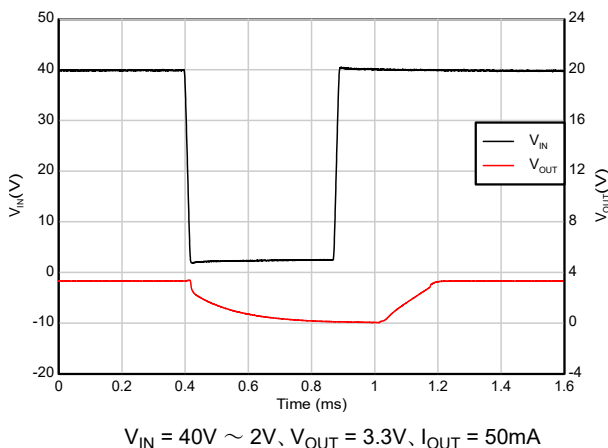
図 7-17. ブラウンアウトからの回復 (40V ~ 2V)
