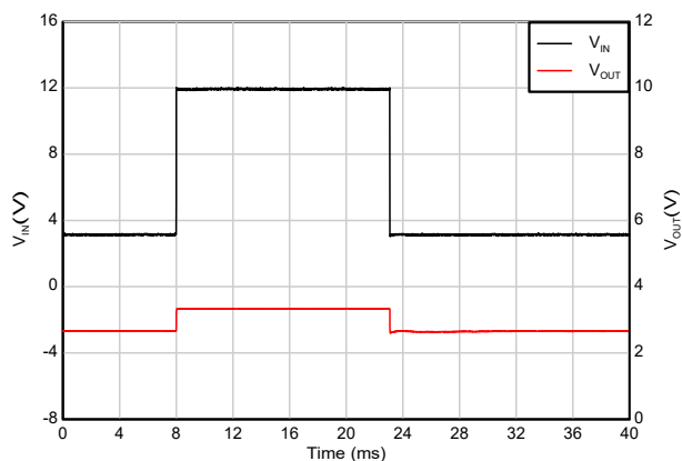
図 5-46. コールドクランク回復
