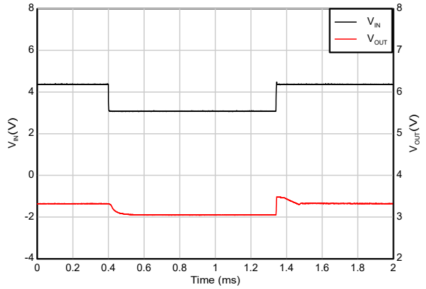
図 5-41. ドロップアウトからの回復 (4.3V 入力 3V 出力)
