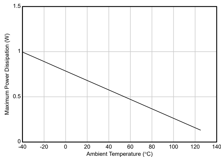
図 7-2. TPS7E82-Q1 (DBV) 許容消費電力
