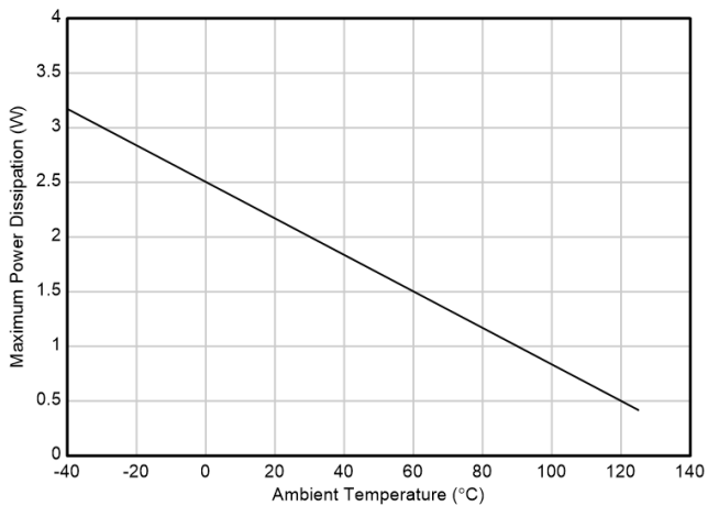
図 7-4. TPS7E82-Q1 (DGN) 許容消費電力
