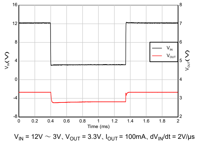
図 5-44. ドロップアウトからの回復 (12V 入力 3V 出力)
