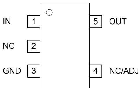
図 4-4. DBV パッケージ、A バージョン (固定/可変)、5 ピン W SOT-23 (上面図)
