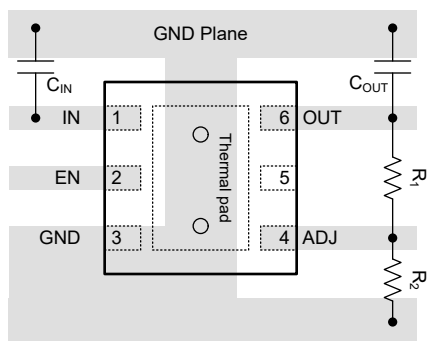
図 7-20. TPS7E82-Q1 DRV パッケージのレイアウト例
