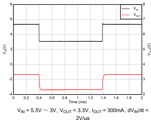
図 7-15. ドロップアウトからの回復 (5.3V 入力 3V 出力)
