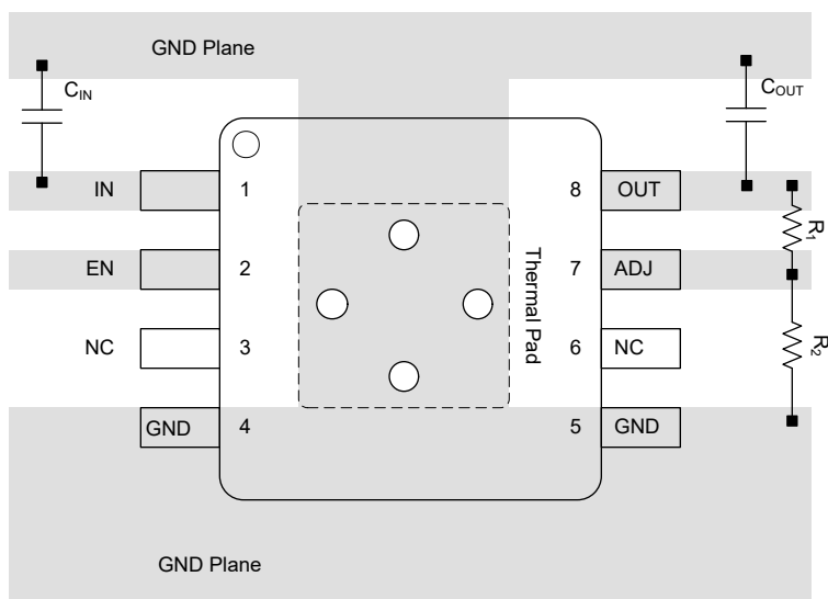
図 7-21. TPS7E82-Q1 DGN パッケージのレイアウト例
