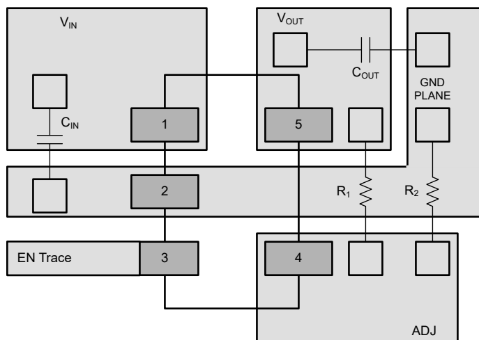
図 7-18. TPS7E82-Q1 (EN 付き) DBV パッケージのレイアウト例
