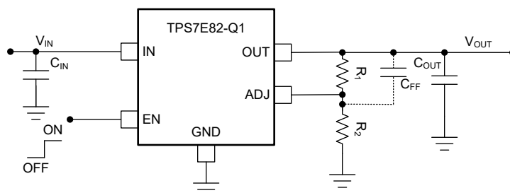
図 7-6. TPS7E82-Q1 の可変 LDO レギュレータのプログラミング
