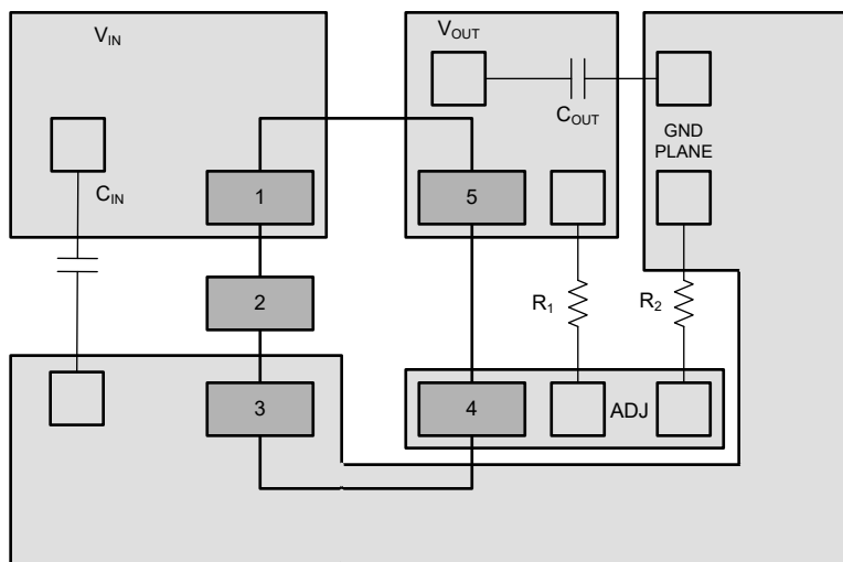
図 7-19. TPS7E82-Q1 (EN なし) DBV パッケージのレイアウト例
