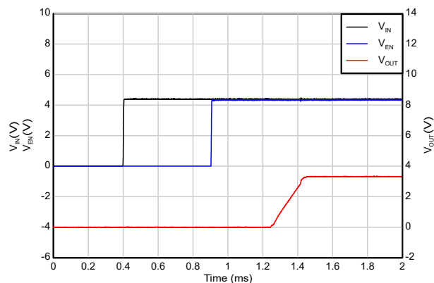
図 5-31. シーケンスによる起動 ( V_{IN} 後の EN)
