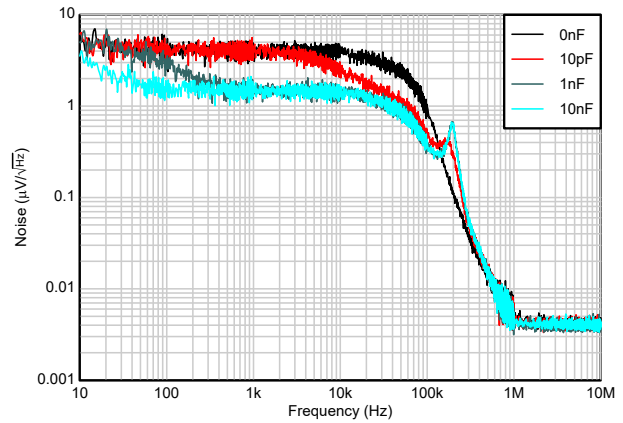
図 5-26. ノイズと C_{FF} との関係
