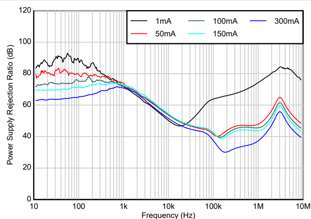
図 5-19. PSRR と I_{OUT} との関係
