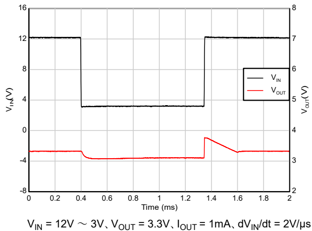
図 5-43. ドロップアウトからの回復 (12V 入力 3V 出力)
