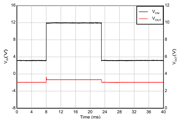
図 5-45. コールドクランク回復
