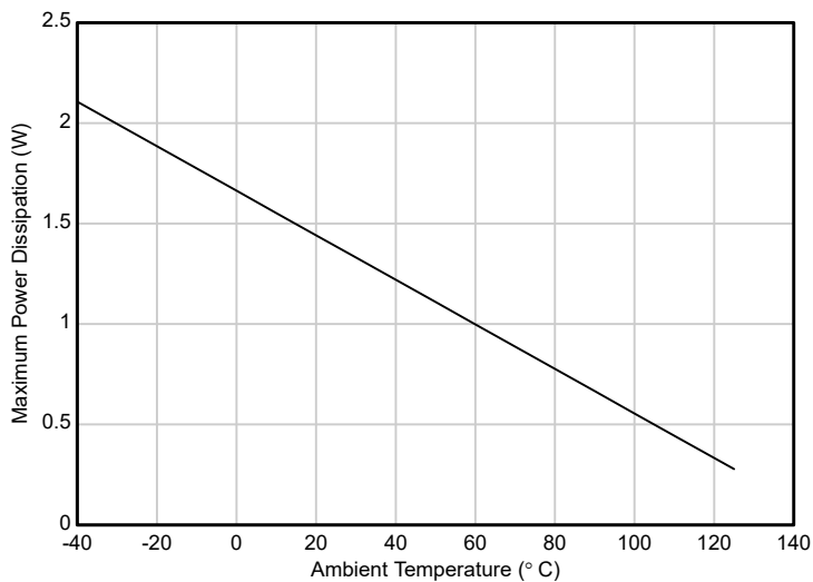
図 7-3. TPS7E82-Q1 (DRV) 許容消費電力
