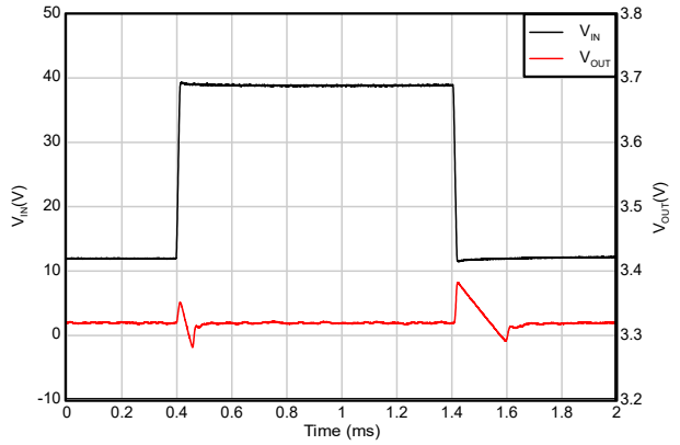
図 5-37. ライン過渡応答 (12V ~ 40V)
