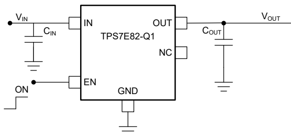
図 7-5. TPS7E82-Q1 代表的なアプリケーションの回路 (固定電圧バージョン)
