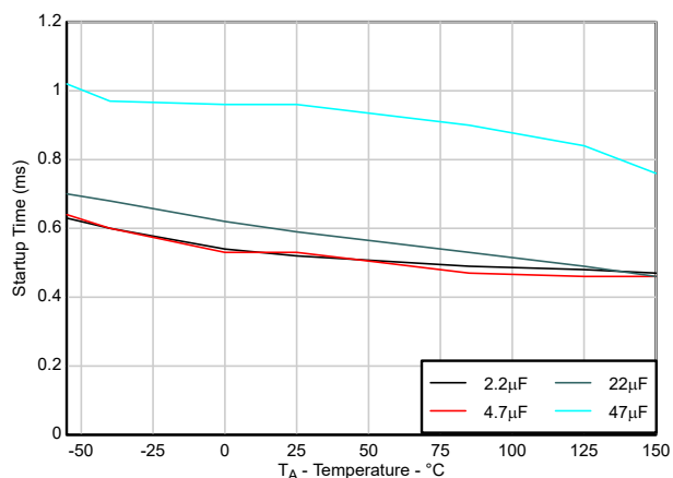
図 5-18. スタートアップタイムと C_{OUT} との関係
