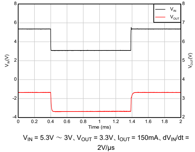
図 5-42. ドロップアウトからの回復 (5.3V 入力 3V 出力)
