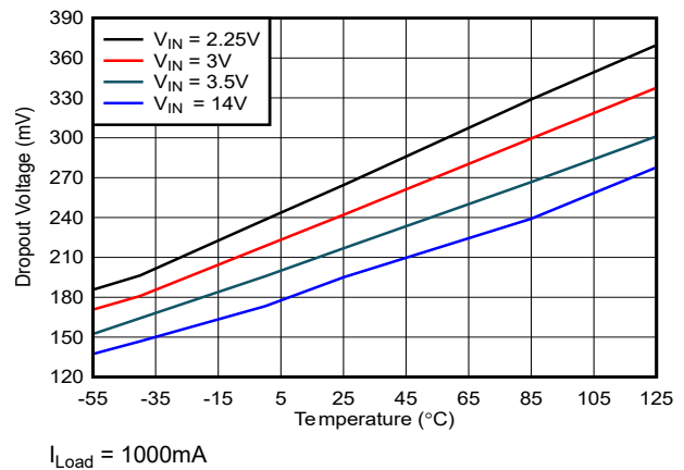
図 6-4. ドロップアウト電圧 vs 温度
