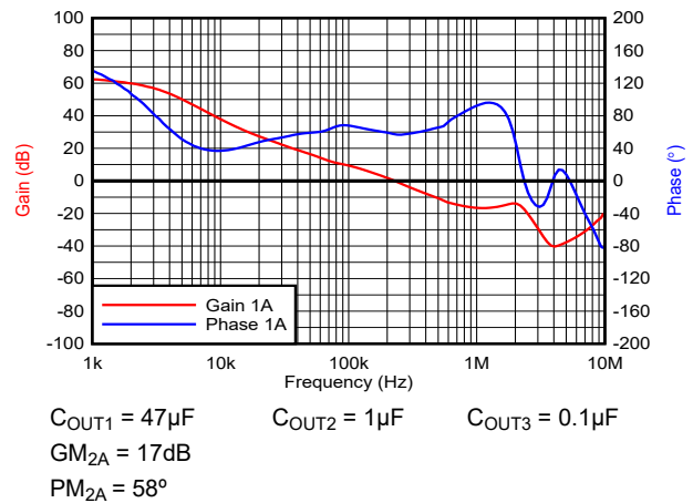
図 6-16. ゲインおよび位相マージンと周波数との関係 (ボード線図)
