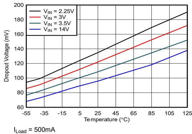
図 6-5. ドロップアウト電圧 vs 温度
