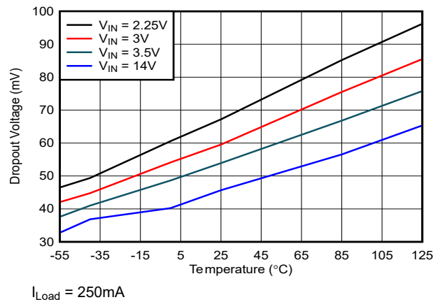
図 6-6. ドロップアウト電圧 vs 温度
