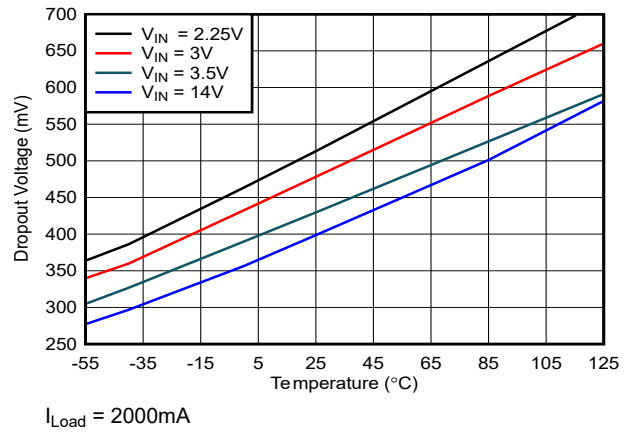
図 6-2. ドロップアウト電圧 vs 温度
