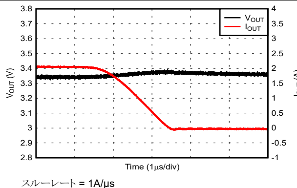
図 6-24. V_{OUT} = 5V の条件で、負荷ステップは 2A から 0A
