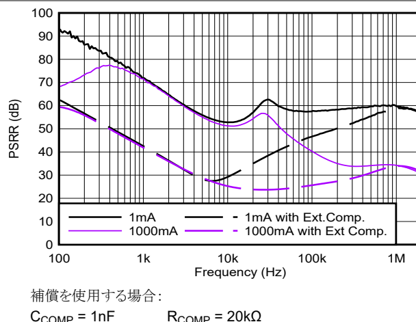
図 6-22. PSRR と周波数との関係、外部補償の比較
