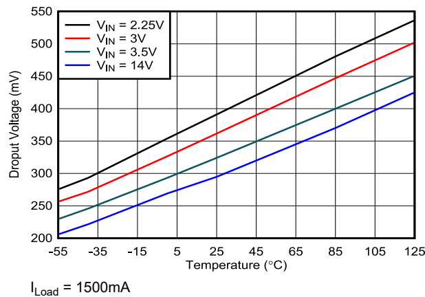
図 6-3. ドロップアウト電圧 vs 温度
