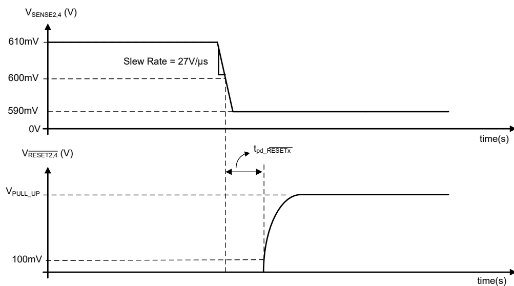
図 7-6. TPS7H31x4 (オープン ドレイン) の \overline{\text{RESET2}} および \overline{\text{RESET4}} の伝搬遅延 ( t_{\text{pd\_RESETx}} ) 時間測定
