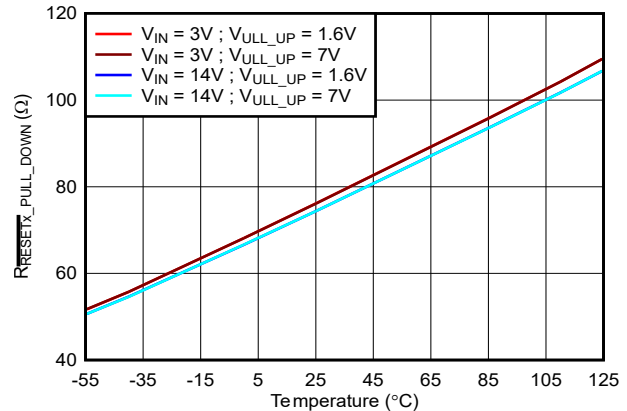
図 6-34. TPS7H3124 で I_{LOAD} = 2mA の条件における RESET1 プルダウン抵抗と V_{PULL\_UP} および V_{IN} 全体の温度との関係
