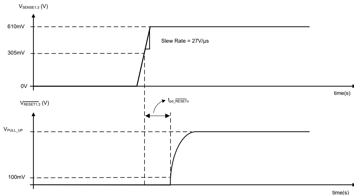
図 7-5. TPS7H31x4 (オープン ドレイン) の \overline{\text{RESET1}} および \overline{\text{RESET3}} の伝搬遅延 ( t_{\text{pd\_RESETx}} ) 時間測定
