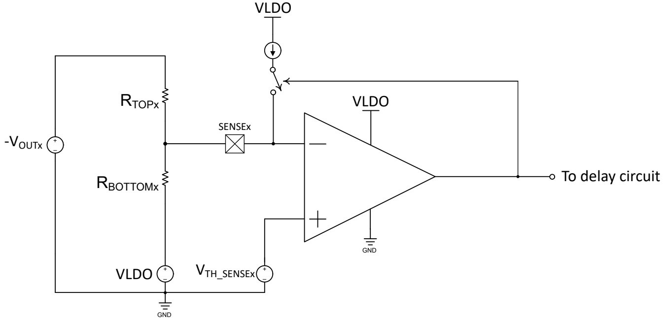
図 9-4. VLDO を使用した TPS7H3xx4 の負電圧監視
