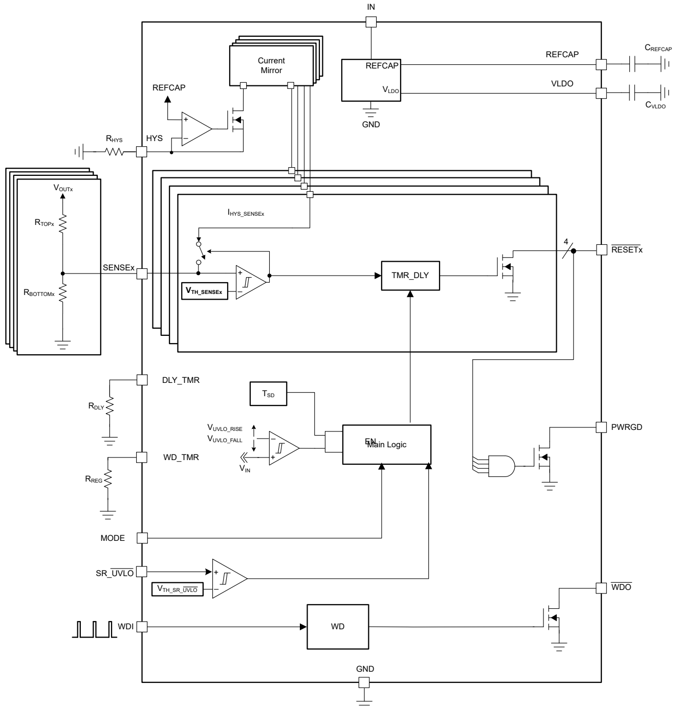
図 8-1. TPS7H30x4 のブロック図 (プッシュプル出力)
