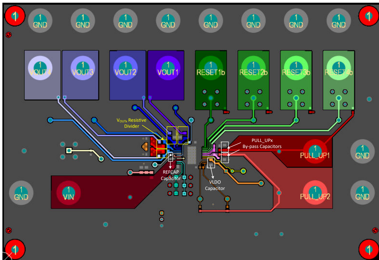
図 9-5. プリント基板のレイアウト例：上層
