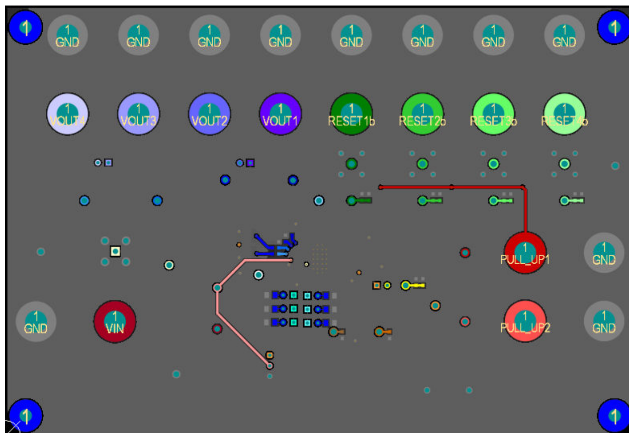
図 9-6. プリント基板のレイアウト例：下層
