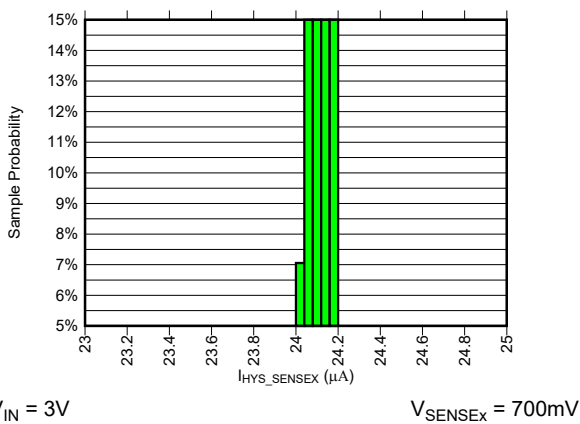
図 6-11. I_{HYS\_SENSEx} 電流分布 (温度 25^{\circ}C )
