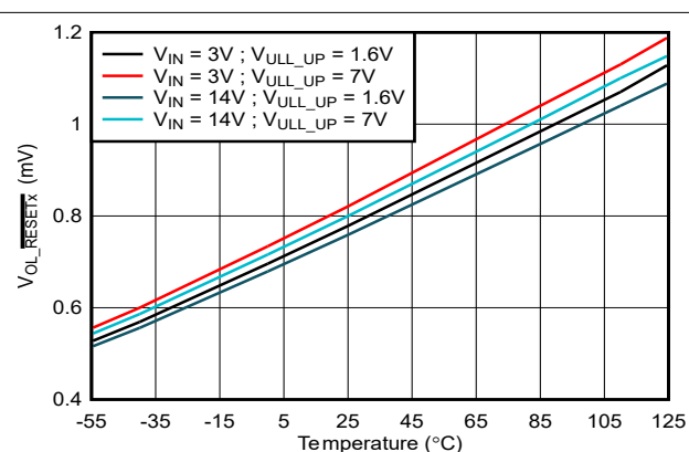
図 6-36. TPS7H3124 で I_{LOAD} = 10mA の条件における RESET1 VOL 電圧と V_{PULL\_UP} および V_{IN} 全体における温度との関係
