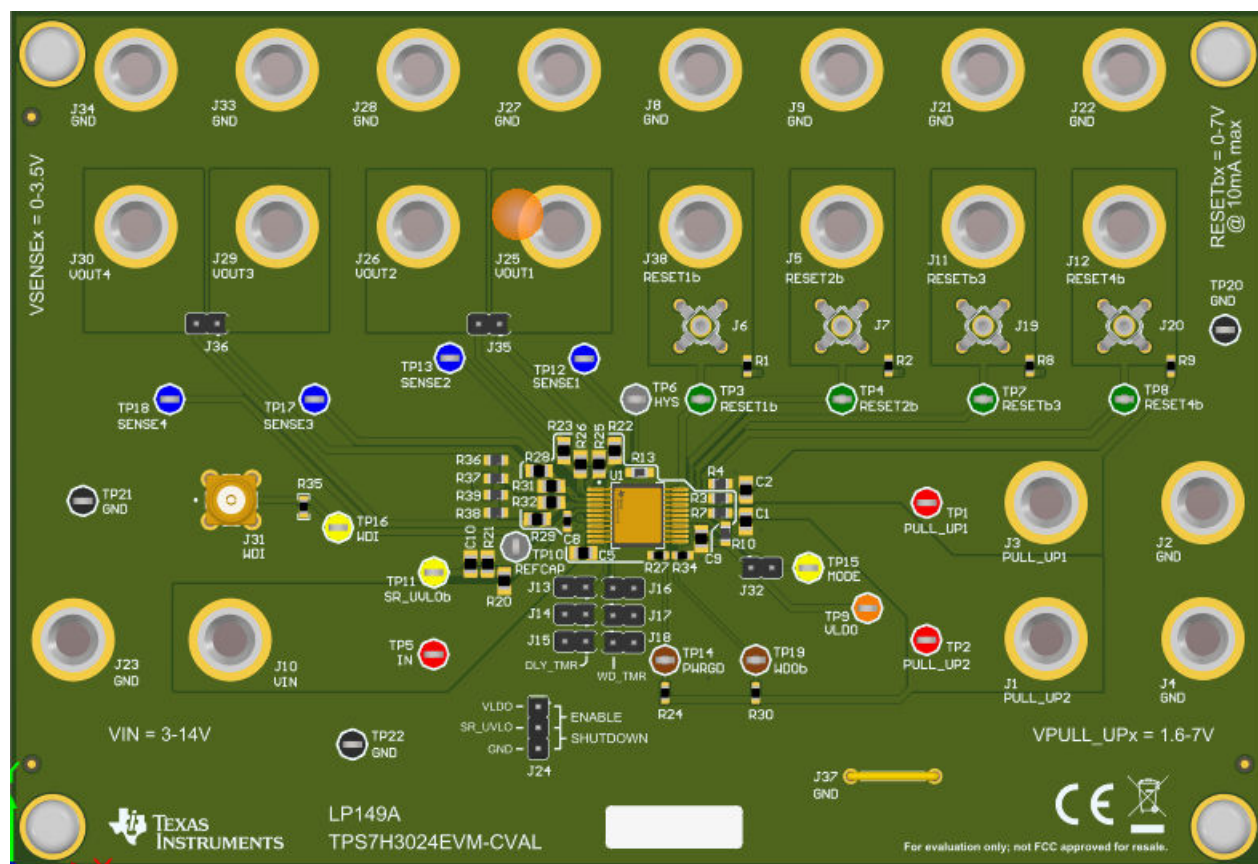
図 9-7. プリント基板のレイアウト例：最上層の 3D ビュー
