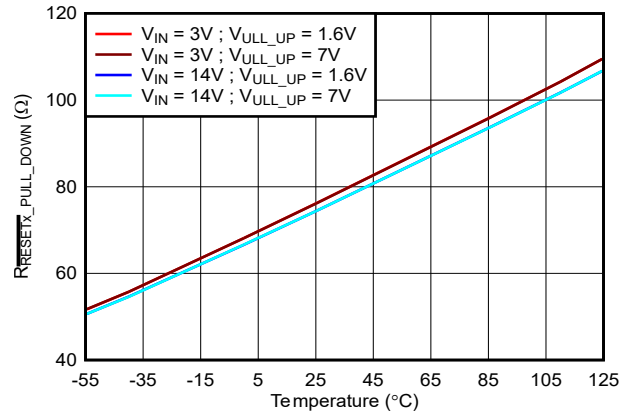
図 6-34. TPS7H3124 で I_{LOAD} = 2mA の条件における RESET1 プルダウ抵抗と V_{PULL\_UP} および V_{IN} 全体の温度との関係
