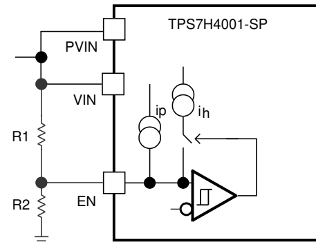
8-3. Adjustable VIN and PVIN UVLO
