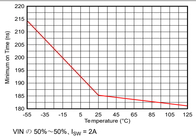
図 7-48. 最小オン時間と温度との関係
