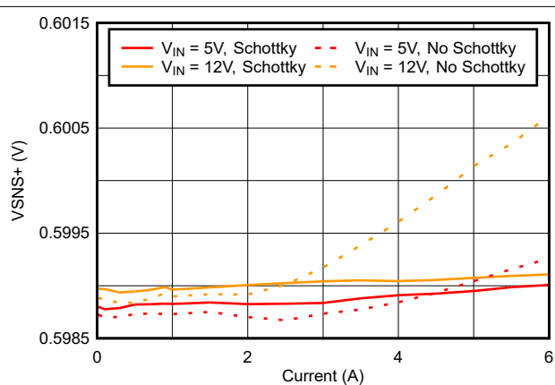
図 7-32. 1MHz での VSNS+ と出力電流の関係
