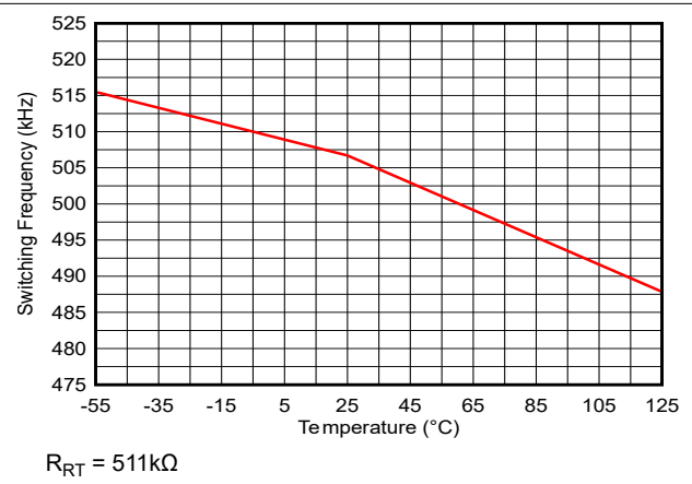
図 7-44. スイッチング周波数と温度との関係
