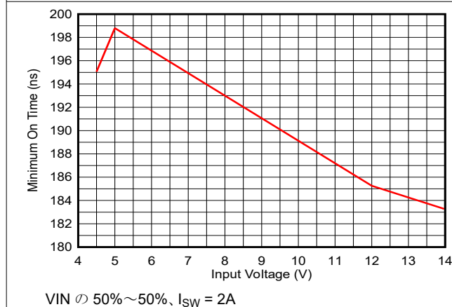
図 7-47. 最小オン時間と入力電圧との関係
