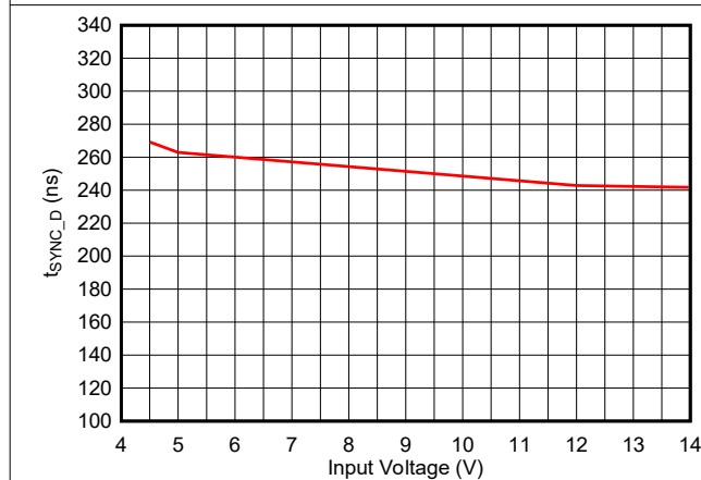
図 7-45. SYNC1 から SW への遅延と入力電圧との関係
