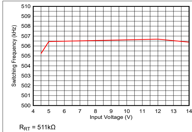
図 7-43. スイッチング周波数と入力電圧との関係
