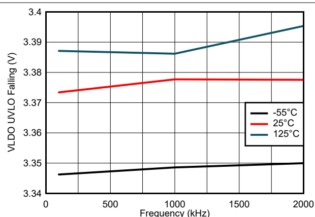
図 7-6. VLDO UVLO Falling Variation
