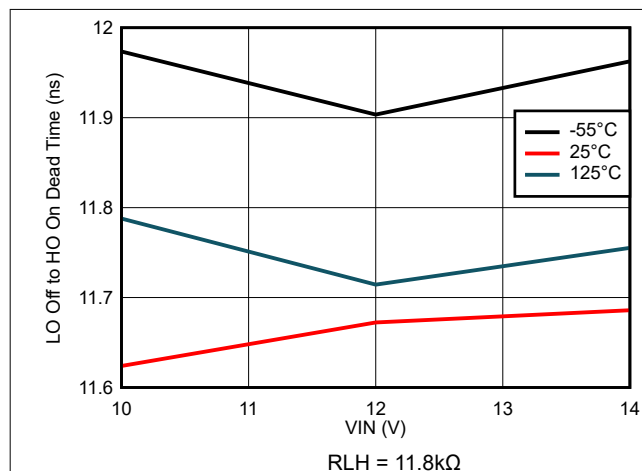
図 7-31. LO オフから HO オンのデッドタイムと VIN 電圧との関係
