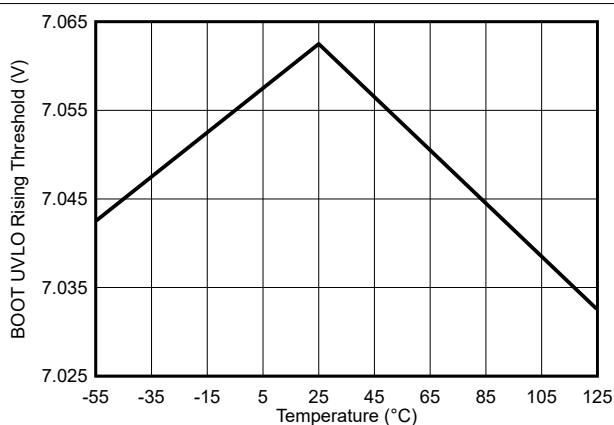
図 7-28. BOOT UVLO 立ち上がりスレッシュォルドと温度の関係
