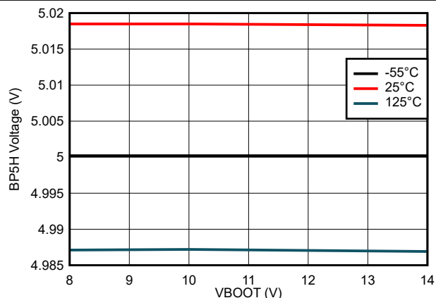
図 7-2. BP5H 出力電圧と BOOT 電圧との関係
