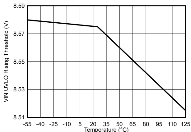
図 7-26. VIN UVLO 立ち上がりスレッシュォルドと温度の関係
