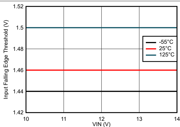
図 7-17. 入力立ち下がりエッジスレッショルドと VIN 電圧との関係
