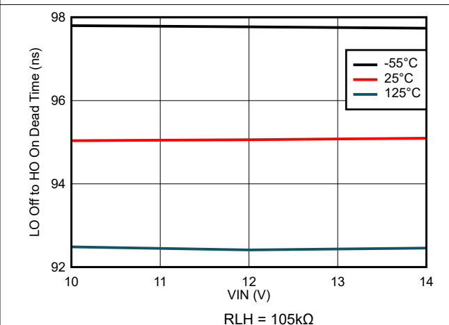
図 7-34. LO オフから HO オンのデッドタイムと VIN 電圧との関係
