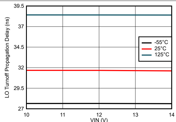
図 7-3. LO ターンオフ伝搬遅延と VIN 電圧 (PWM) との関係
