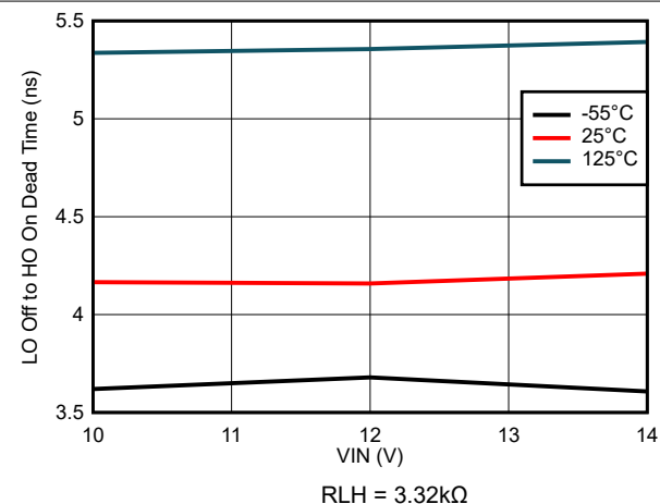
図 7-30. LO オフから HO オンのデッドタイムと VIN 電圧との関係
