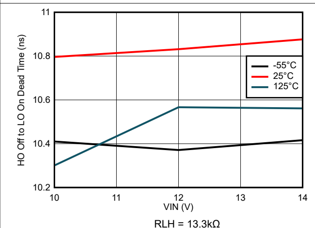
図 7-36. HO オフから LO オンのデッドタイムと VIN 電圧との関係
