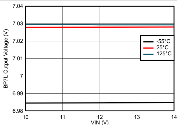
図 7-15. BP7L 出力電圧と VIN 電圧との関係
