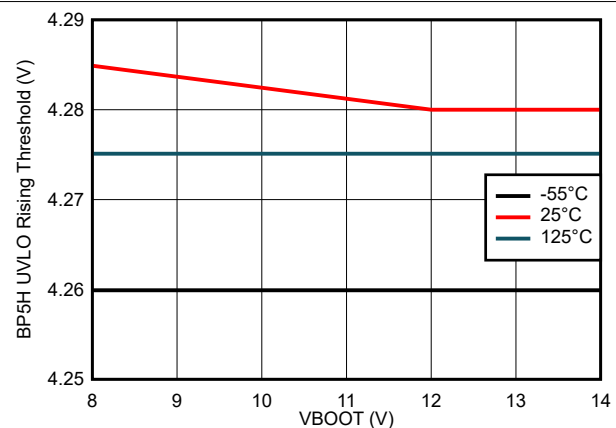
図 7-22. BP5H UVLO 立ち上がりスレッシュホールドと BOOT 電圧との関係
