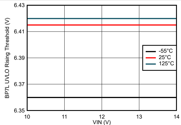
図 7-24. BP7L UVLO 立ち上がりスレッシュホールドと VIN 電圧との関係
