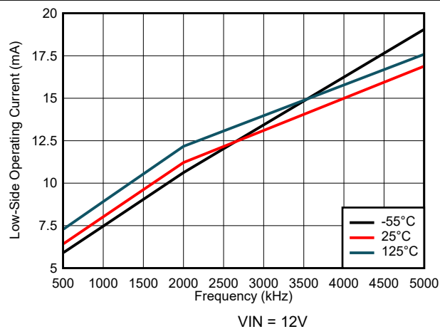
図 7-43. ローサイド動作電流と周波数との関係 (PWM)
