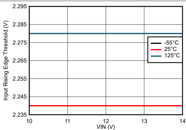
図 7-16. 入力立ち上がりエッジスレッショルドと VIN 電圧との関係
