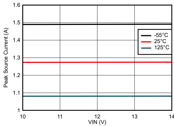
図 7-9. ピークソース電流と VIN 電圧との関係
