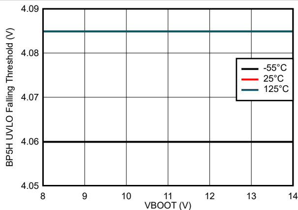
図 7-23. BP5H UVLO 立ち下がりスレッシュホールドと BOOT 電圧との関係
