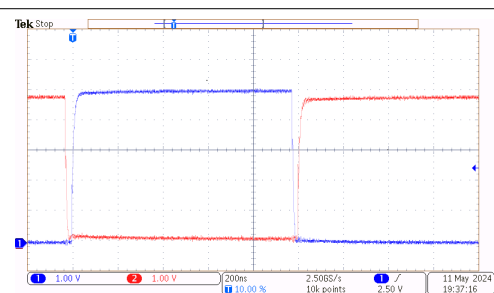
図 9-3. TPS7H6005EVM、PWM モードの 500kHz HO (青) および LO (赤) ゲートドライバ出力
