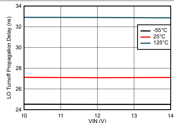
図 7-4. LO ターンオフ伝搬遅延と VIN 電圧 (IIM) との関係
