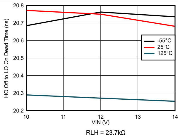
図 7-37. HO オフから LO オンのデッドタイムと VIN 電圧との関係
