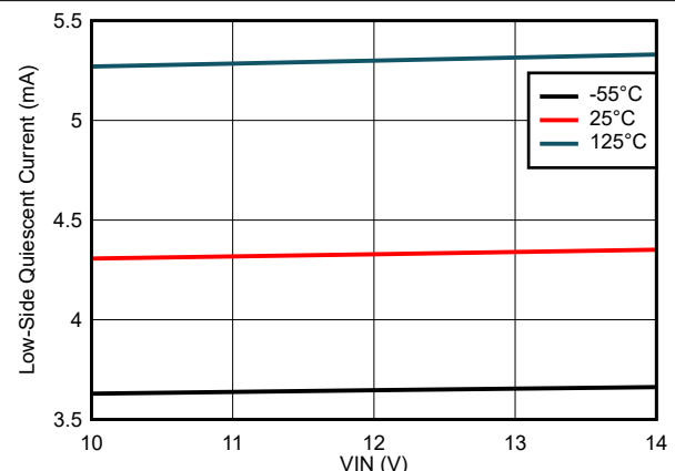
図 7-40. ローサイド静止電流と VIN 電圧との関係
