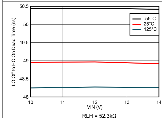
図 7-33. LO オフから HO オンのデッドタイムと VIN 電圧との関係
