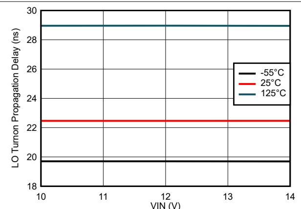
図 7-5. LO ターンオン伝搬遅延と VIN 電圧 (IIM) との関係
