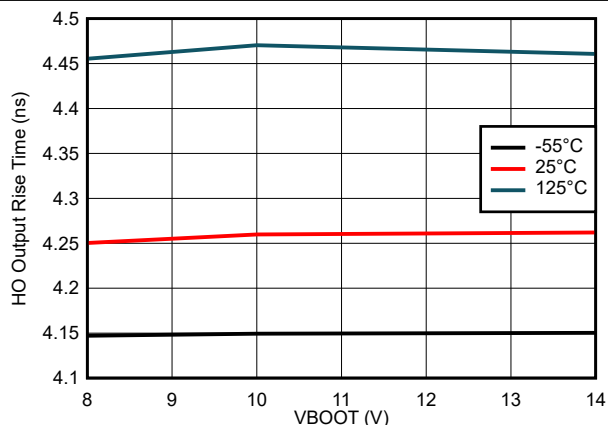
図 7-14. HO 出力立ち上がり時間とブート電圧との関係
