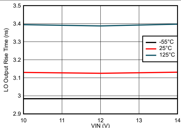
図 7-13. LO 出力立ち上がり時間と VIN 電圧との関係
