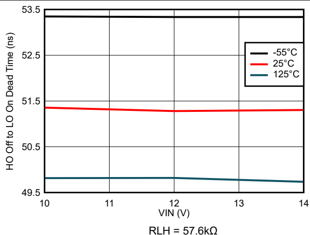
図 7-38. HO オフから LO オンのデッドタイムと VIN 電圧との関係
