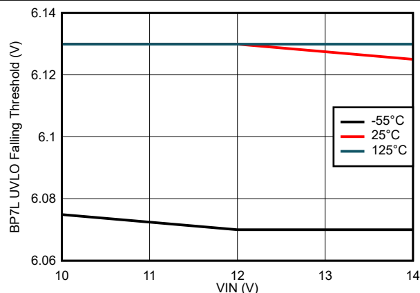
図 7-25. BP7L UVLO 立ち下がリスレッシュォルドと VIN 電圧との関係
