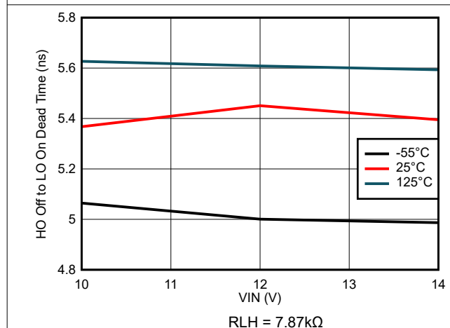
図 7-35. HO オフから LO オンのデッドタイムと VIN 電圧との関係
