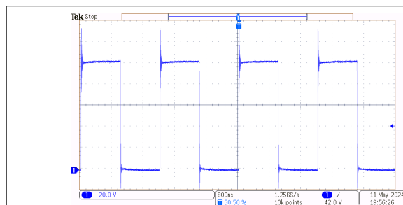
図 9-2. TPS7H6005EVM からの 100V、500kHz のスイッチノード信号
