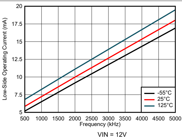
図 7-42. ローサイド動作電流と周波数との関係 (IIM)
