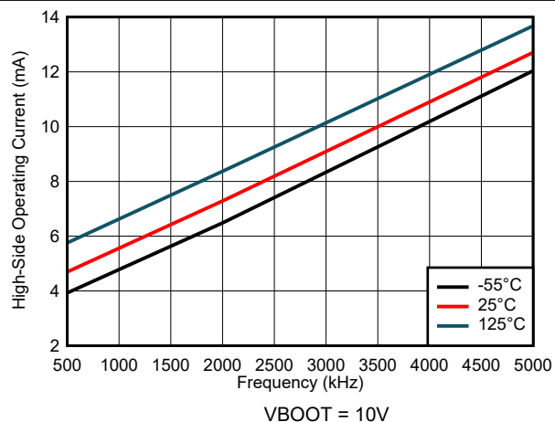
図 7-44. ハイサイド動作電流と周波数との関係 (IIM)
