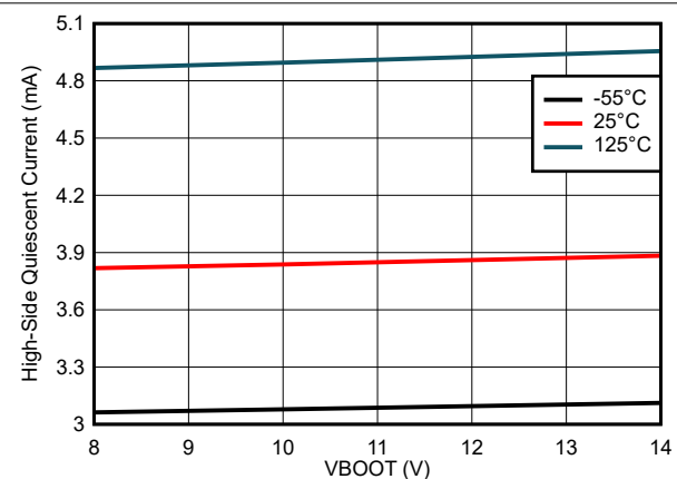
図 7-41. ハイサイド静止電流とブート電圧との関係
