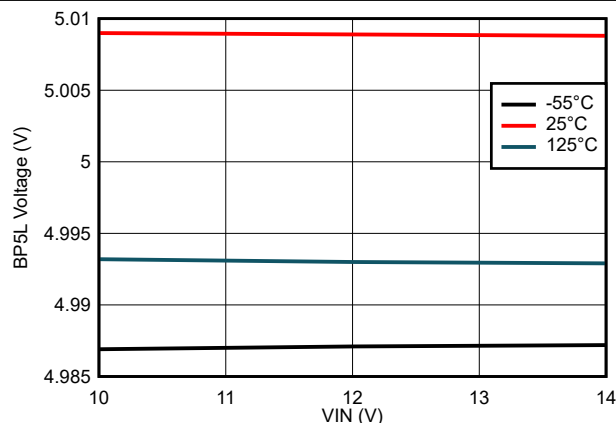
図 7-1. BP5L 出力電圧と VIN 電圧との関係
