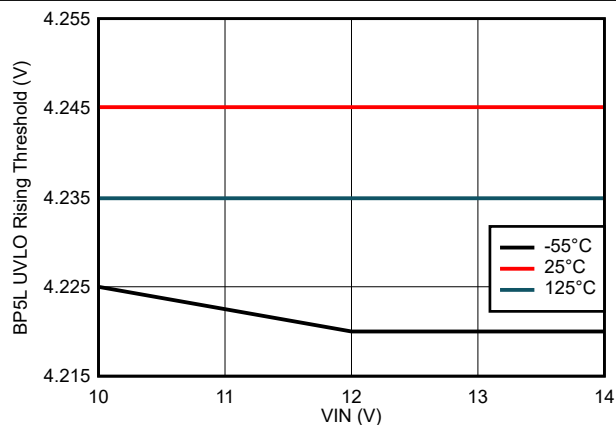
図 7-20. BP5L UVLO 立ち上がりスレッシュホールドと VIN 電圧との関係
