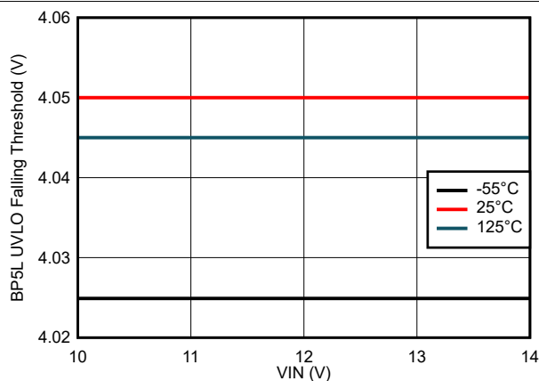
図 7-21. BP5L UVLO 立ち下がりスレッシュホールドと VIN 電圧との関係
