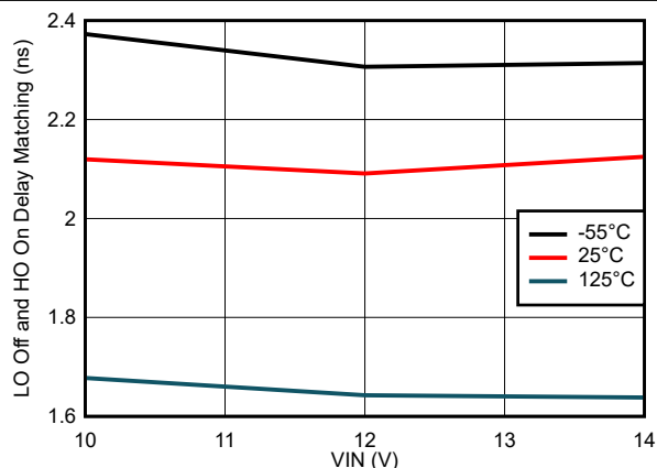
図 7-19. LO オフおよび HO オン遅延マッチングと VIN 電圧との関係
