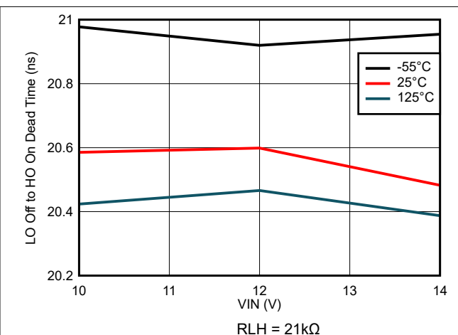
図 7-32. LO オフから HO オンのデッドタイムと VIN 電圧との関係
