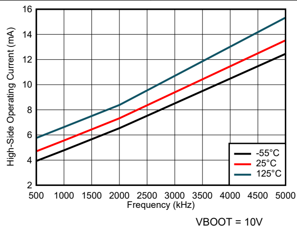
図 7-45. ハイサイド動作電流と周波数との関係 (PWM)
