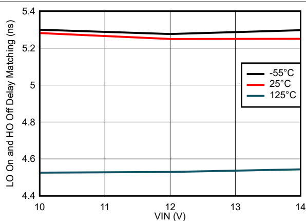
図 7-18. LO オンおよび HO オフ遅延マッチングと VIN 電圧との関係
