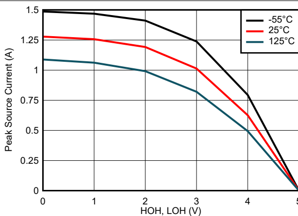
図 7-11. ピークソース電流と出力電圧との関係
