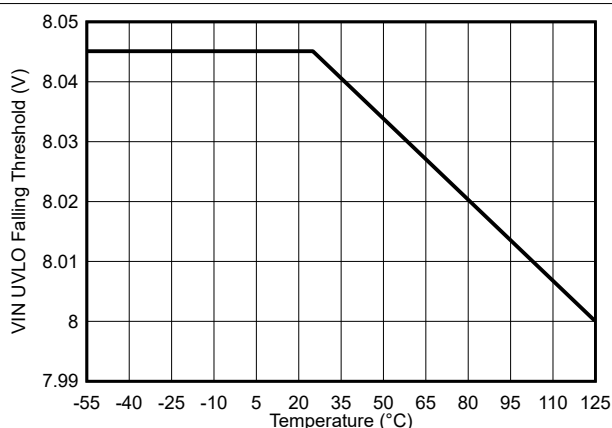
図 7-27. VIN UVLO 立ち上がりスレッシュォルドと温度の関係
