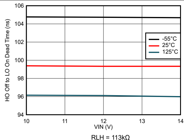
図 7-39. HO オフから LO オンのデッドタイムと VIN 電圧との関係
