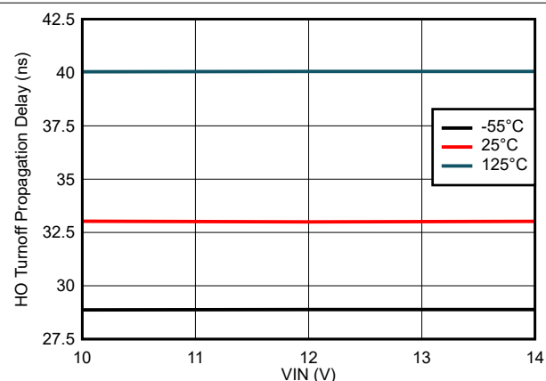
図 7-6. HO ターンオフ伝搬遅延と VIN 電圧 (PWM) との関係
