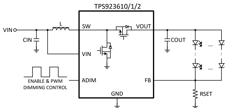
概略回路図
