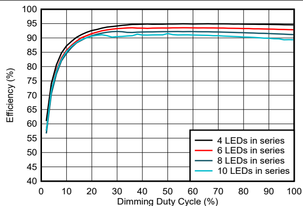
図 6-2. 効率 vs 調光デューティ サイクル
