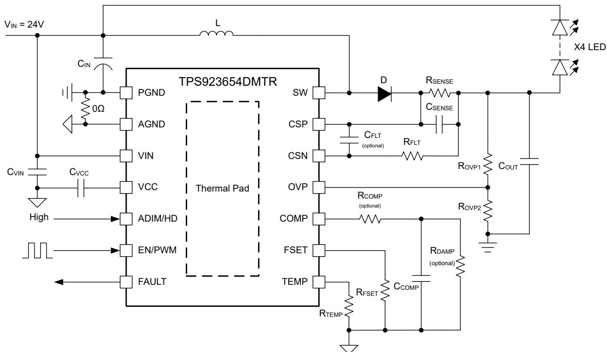
図 8-12. 昇降圧、24V 入力、2A 出力、4 ピース WLED、PWM 調光のリファレンスデザイン
