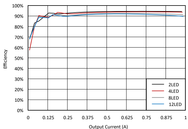
図 6-12. 入力電圧 13V、出力電流 1A 時の効率
