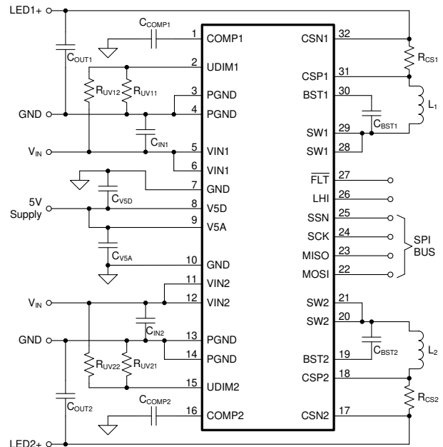
概略回路図
