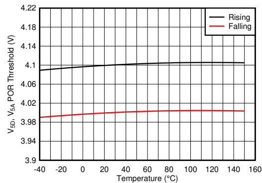
6-6. V_{5D,A} POR Threshold vs Temperature
