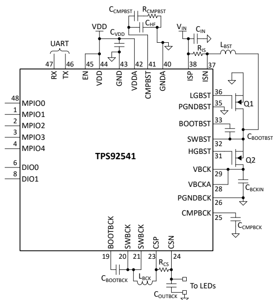
概略回路図
