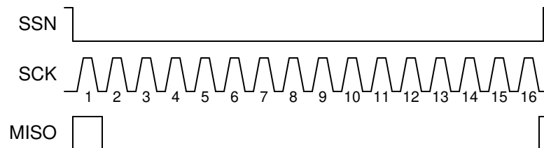
图 7-26. Write Error/POR
