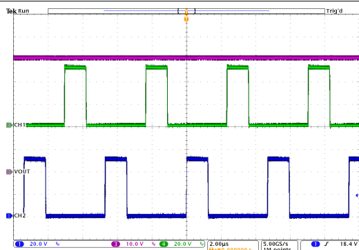
CH1: Phase-1 V_{SW} CH2: Phase-2 V_{SW} CH3: CV Boost V_{OUT}
