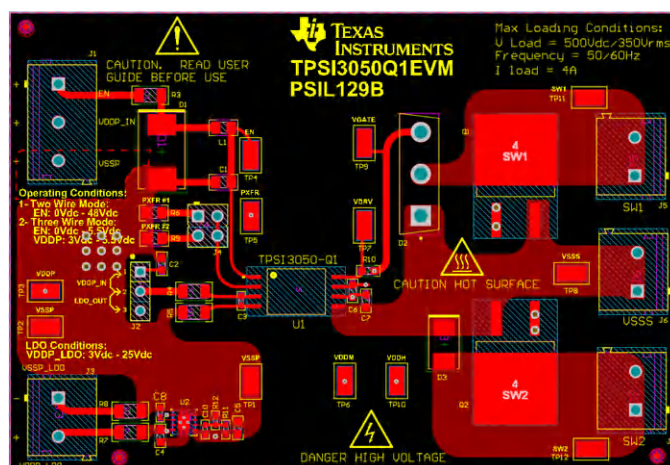
図 9-15. Top Layer
