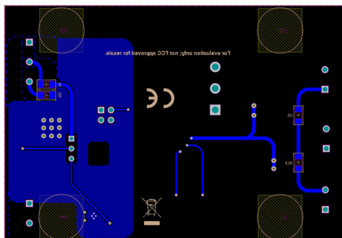
図 9-16. Bottom Layer
