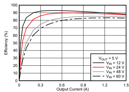
標準的な効率、 V_{OUT} = 5V
