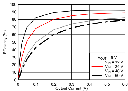
標準的な効率、V OUT = 5V
