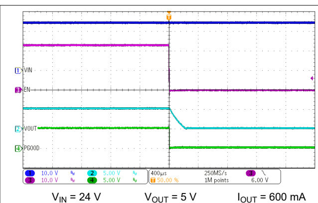
图 8-3. Enable Shutdown Waveforms
