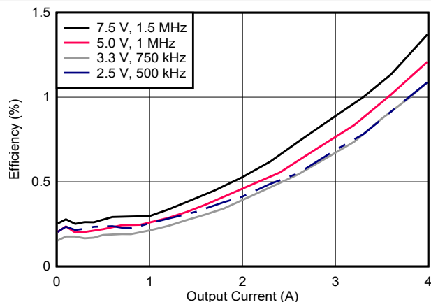
図 7-10. Power Dissipation
