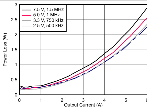
図 7-10. Power Dissipation
