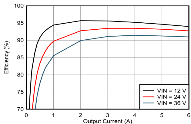
代表的な効率、 V_{OUT} = 5\text{ V} 、 F_{SW} = 1\text{ MHz}
