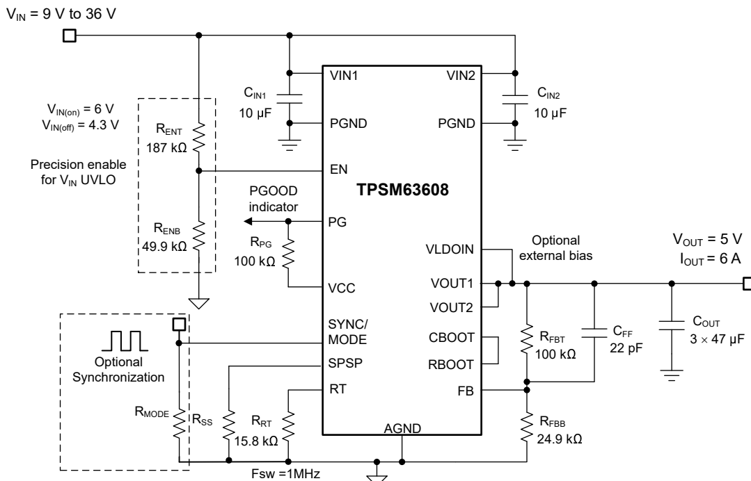
図 9-1. Circuit Schematic
