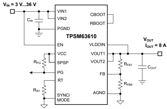
代表的な回路図
