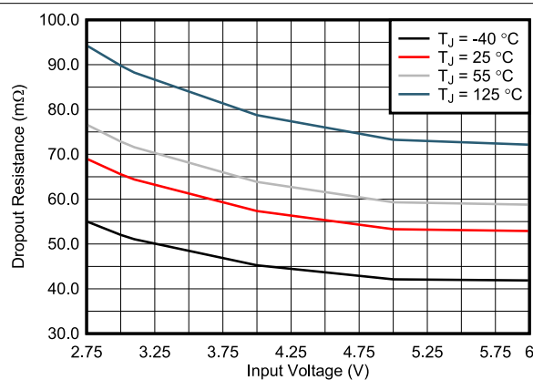
図 6-4. ドロップアウト抵抗
