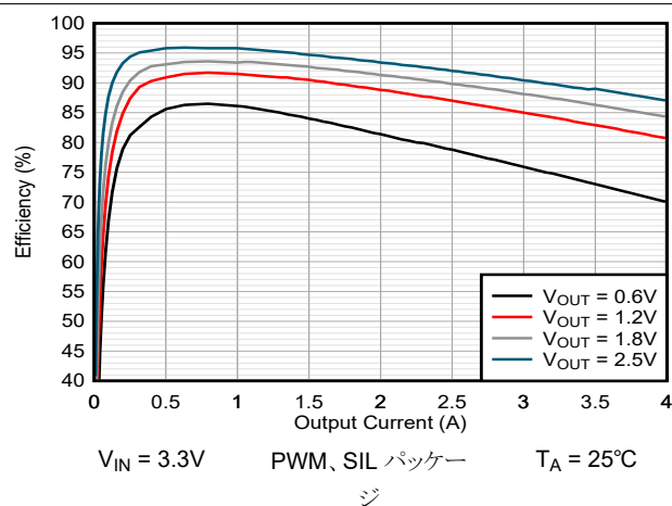
図 9-3. 効率と出力電流との関係
