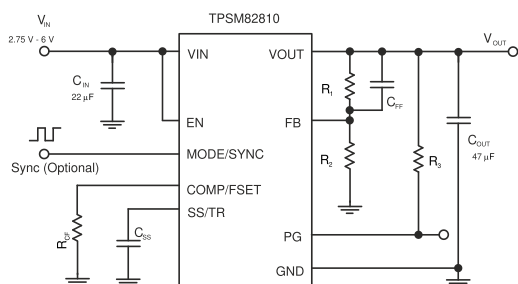
回路図
