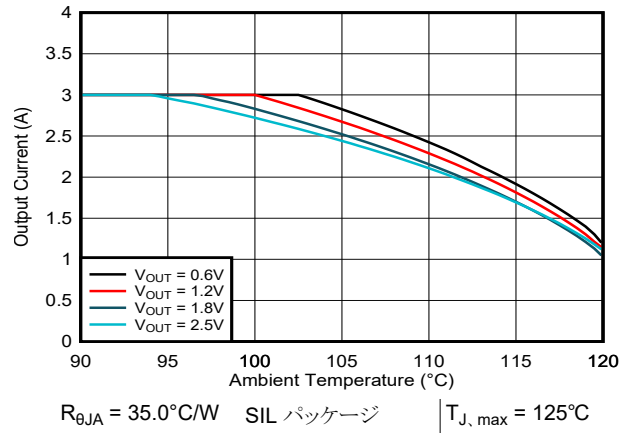
図 9-23. 安全動作領域 V_{IN} = 3.3V
