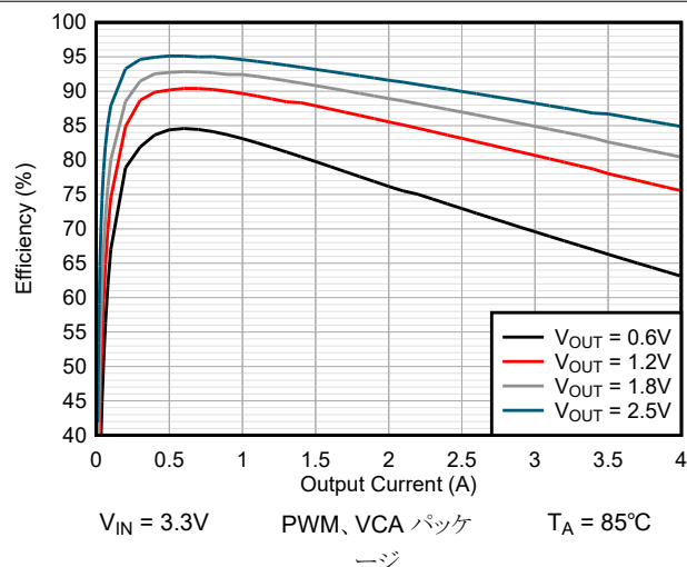
図 9-13. 効率と出力電流との関係
