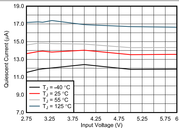
図 6-1. 静止電流
