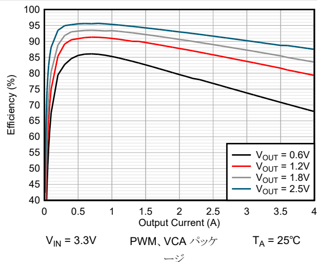
図 9-11. 効率と出力電流との関係
