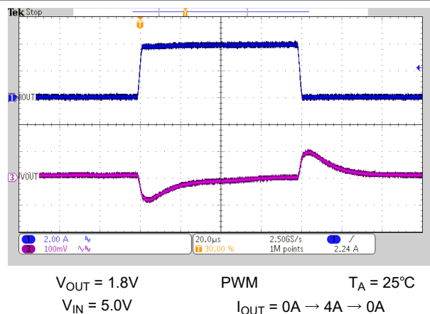
図 9-27. 負荷過渡応答
