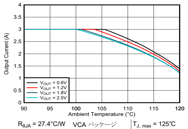
図 9-25. 安全動作領域 V_{IN} = 3.3V
