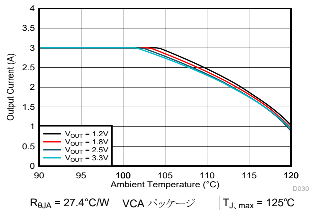
図 9-26. 安全動作領域 V_{IN} = 5.0V
