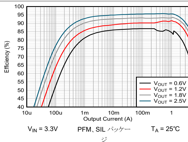
図 9-2. 効率と出力電流との関係
