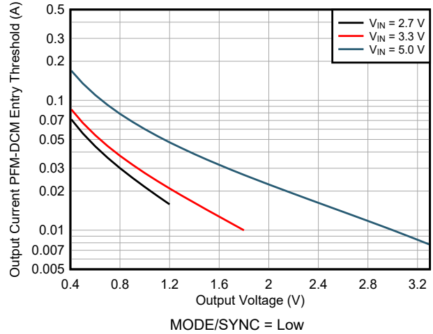
図 7-6. PFM-DCM Entry Threshold TPSM8287A12BAS
