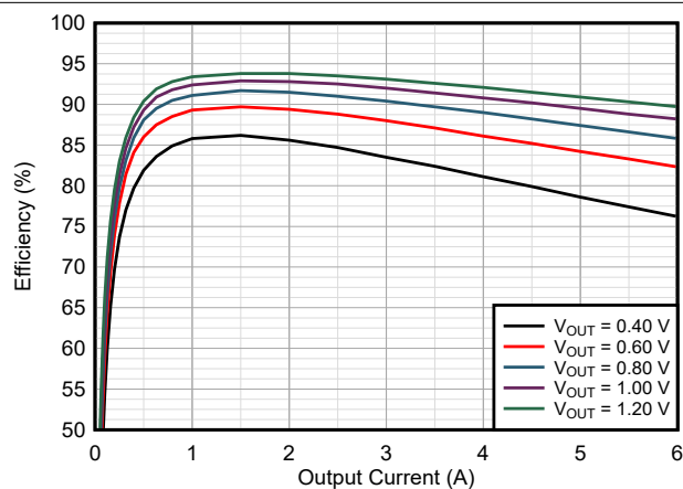
図 9-2. Efficiency TPSM8287A06BAS
