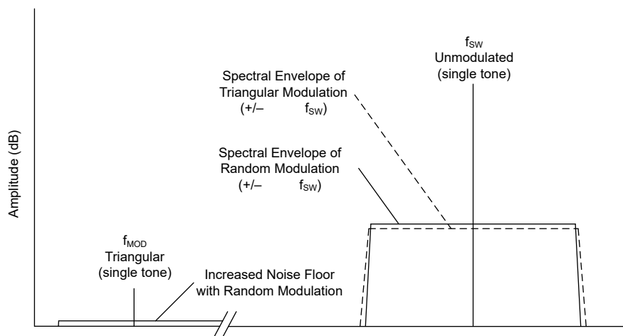
図 6-2. スペクトラム拡散変調
