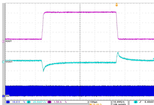
300mA から 4.5A を経て 300mA 12V ~ 3.3V 1μH, 2.2MHz 1 段目の L-C のみ
