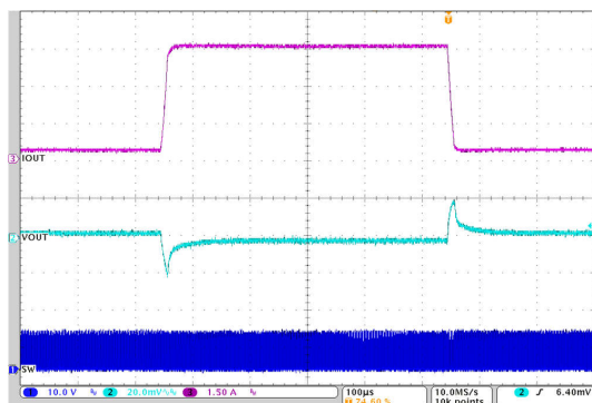
300mA から 4.5A を経て 300mA 12V ~ 1.8V 1μH, 1MHz 1 段目の L-C のみ
