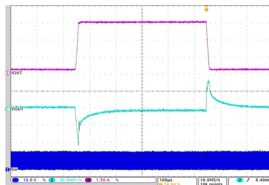
300mA から 4.5A を経て 300mA 12V ~ 3.3V 1μH, 2.2MHz 2 段目の L-C の後
