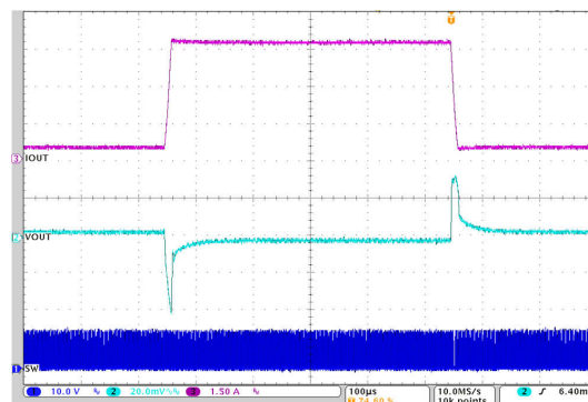
300mA から 4.5A を経て 300mA 12V ~ 1.8V 1μH, 1MHz 2 段目の L-C の後
