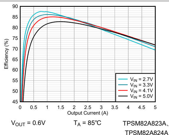
図 8-37. 効率
