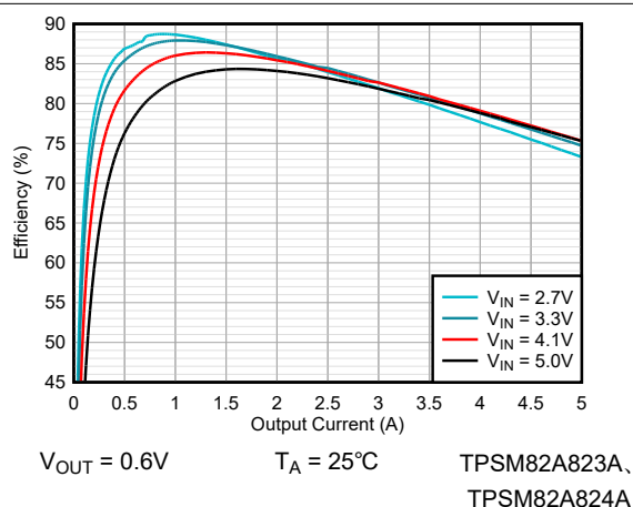
図 8-36. 効率
