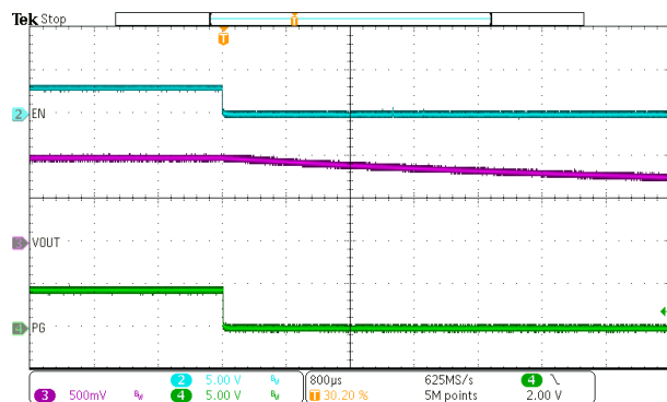
7-10. EN Shutdown No Load
