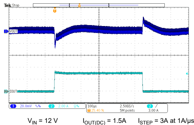
図 7-8. Load Transient
