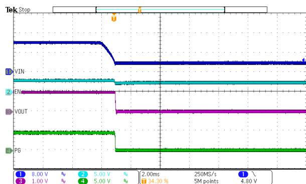
I_{OUT} = 6A 図 7-14. VIN Shutdown
