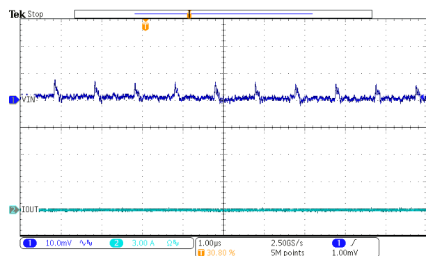
図 7-17. Input Ripple – No Load
