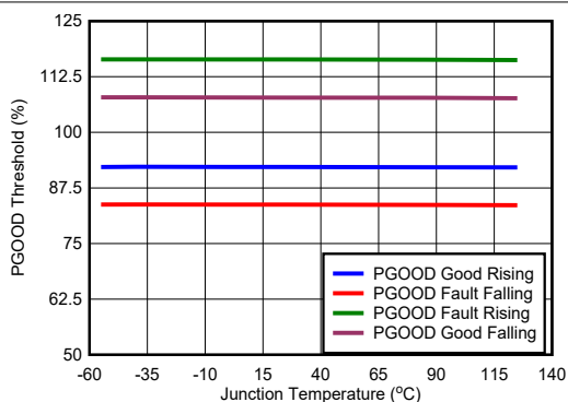
図 5-9. PG Threshold
