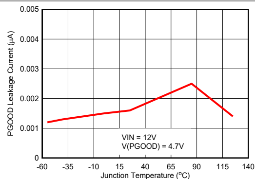
図 5-10. PG Leakage
