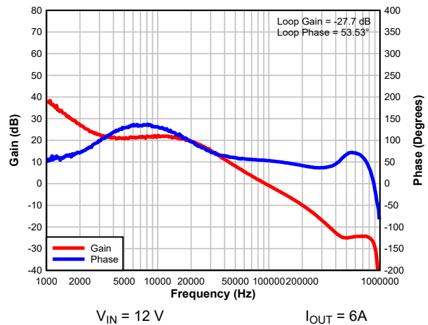
図 7-7. Bode Plot
