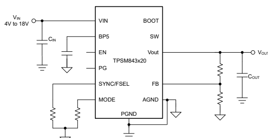
概略回路図
