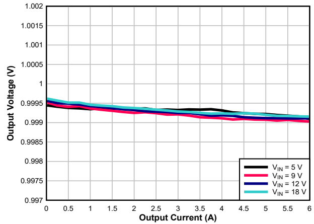
図 7-5. Load Regulation
