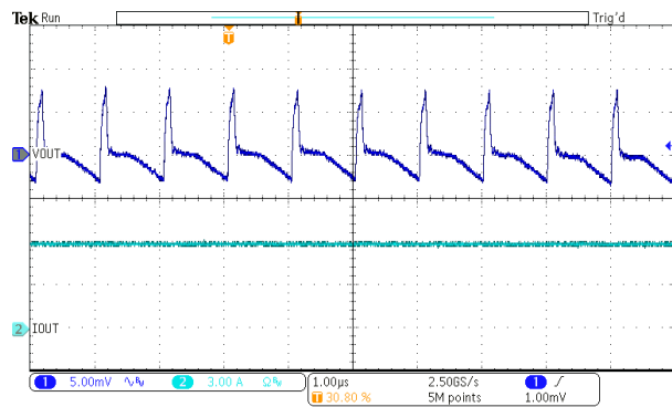
図 7-16. Output Ripple – 6A Load
