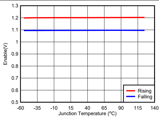
図 5-5. Enable Voltage
