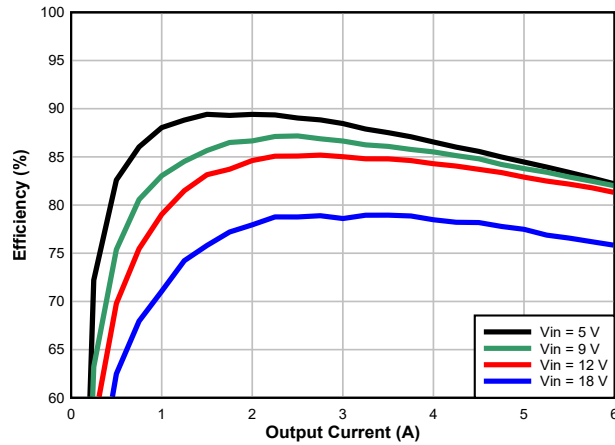
図 7-4. Efficiency
